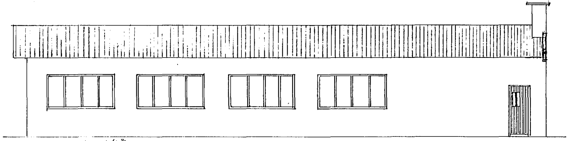
Norð-Vesturhlíð
