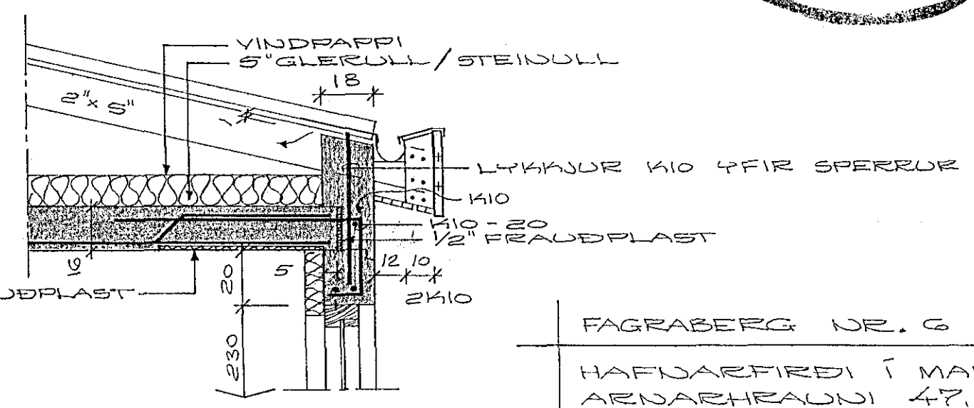
SKURÐUR A, M=1:20
