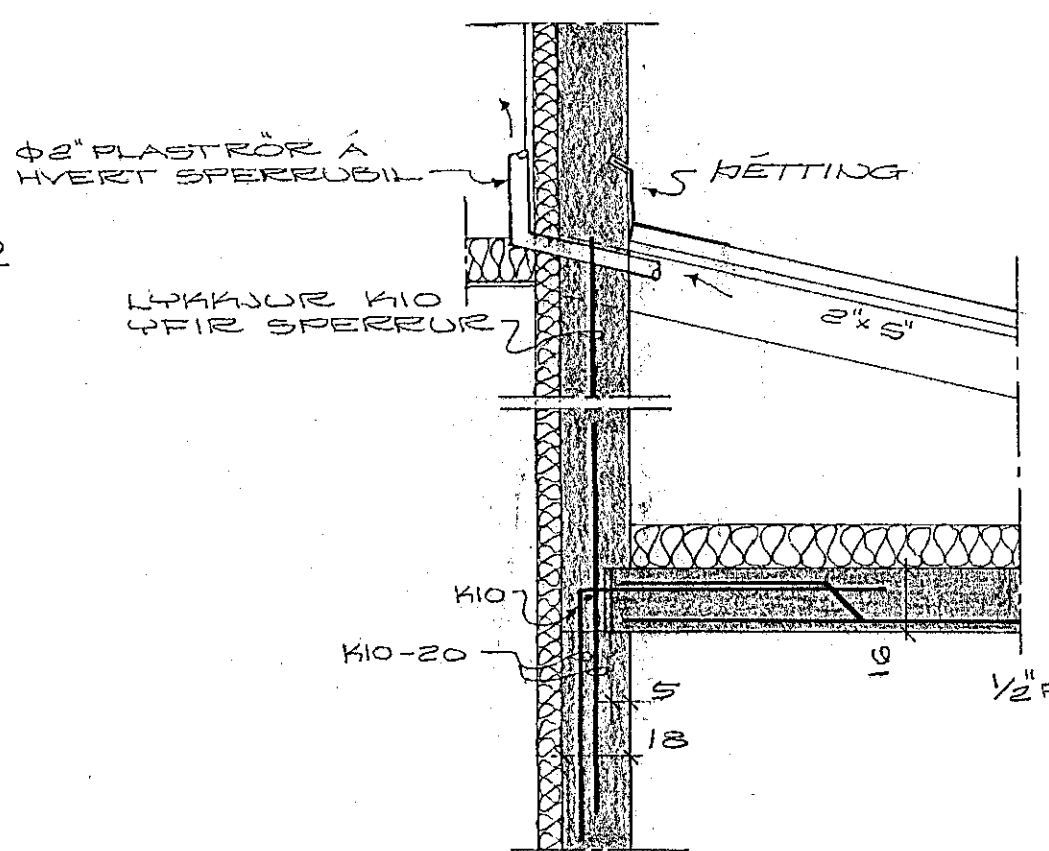
SKURÐUR B, M=1:20
