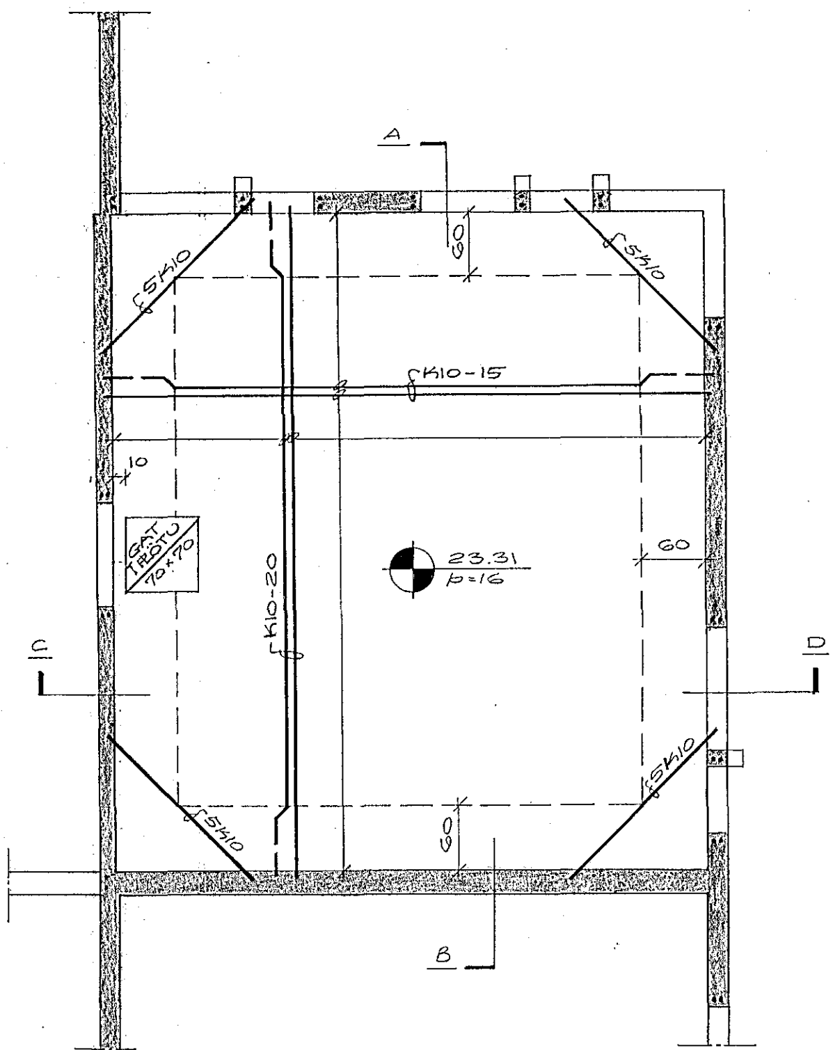
GRUNNUMYND, M=1:50
