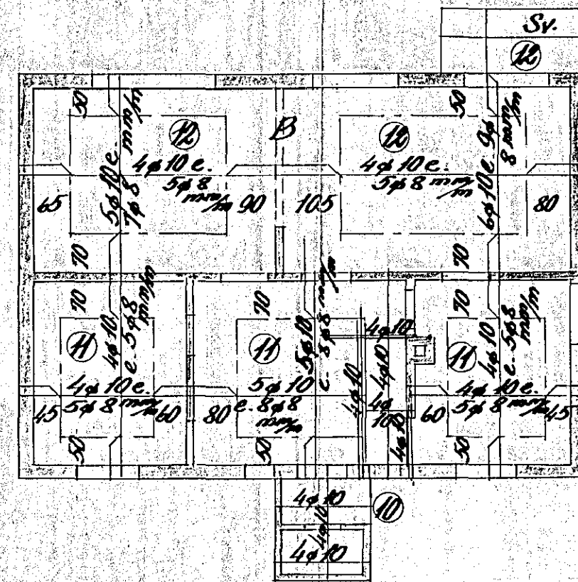
Loft yfir kjallara 1:100
