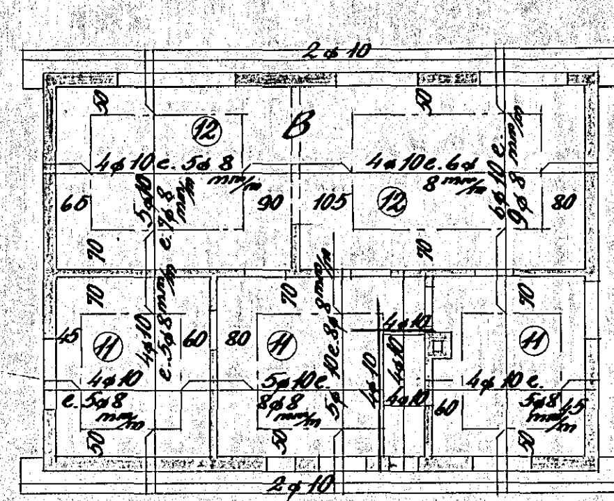
Loft yfir hæð 1:100
