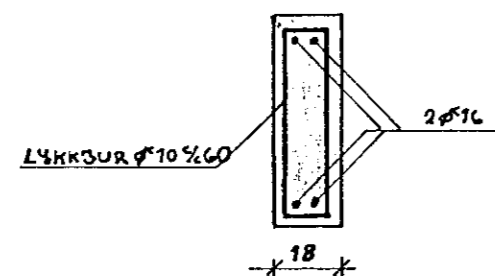
SNIÐ B-B 1:20
