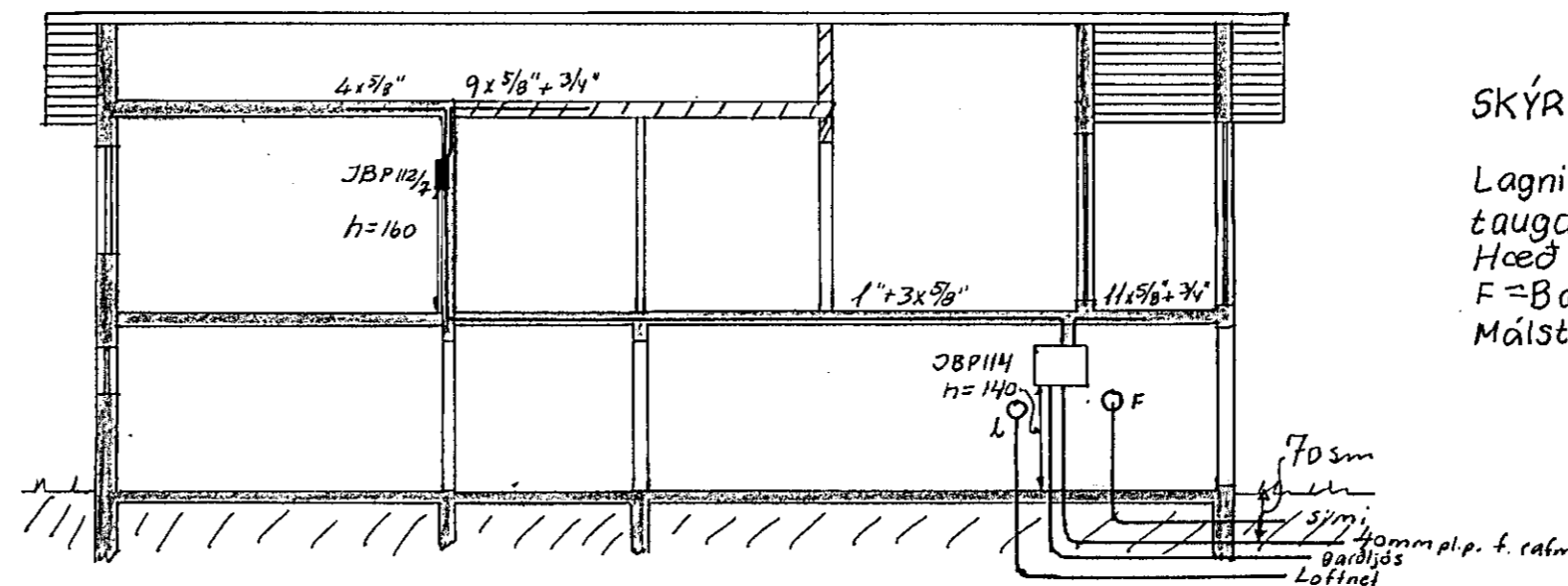
Sníð A-A í Inntak M. 1:100
