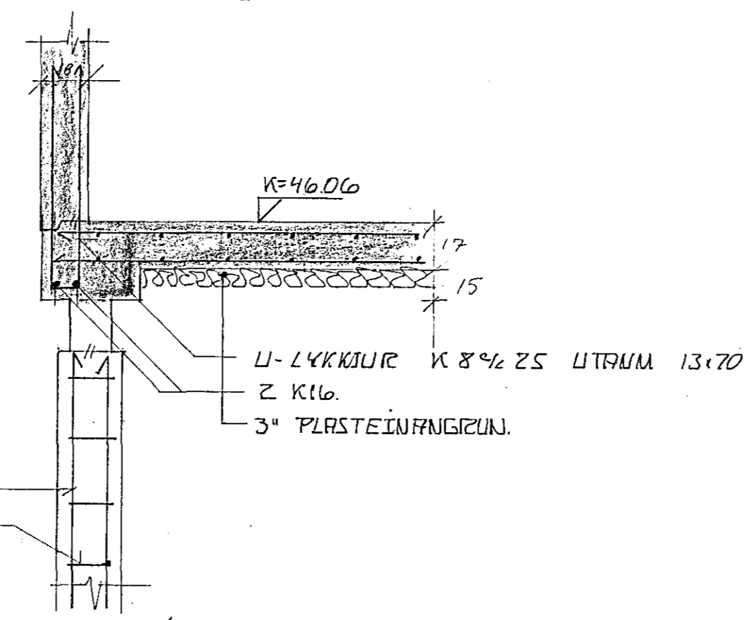
SÚLA SI M.1:20
