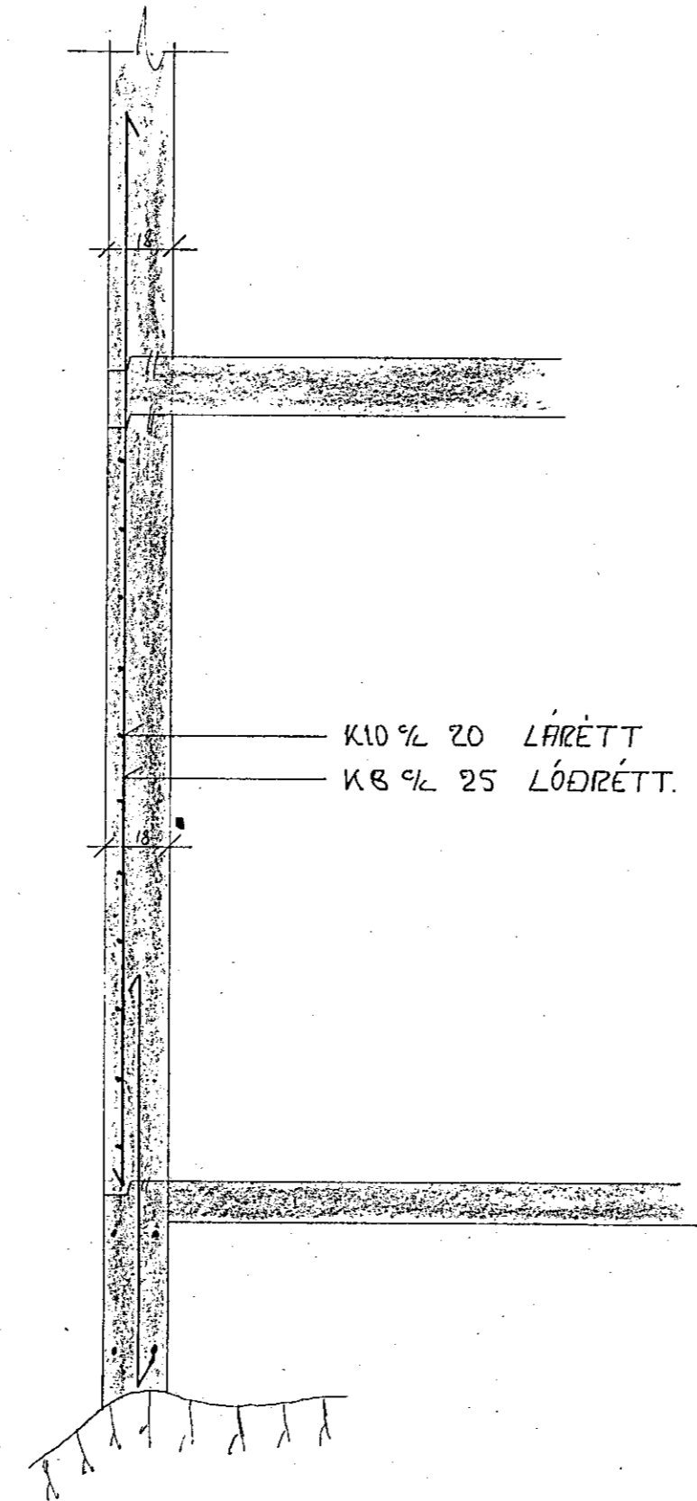
SNÍÐ B-B M.1:20
