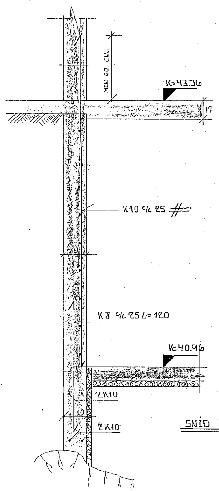
SNÍÐ G-G M.1:20
