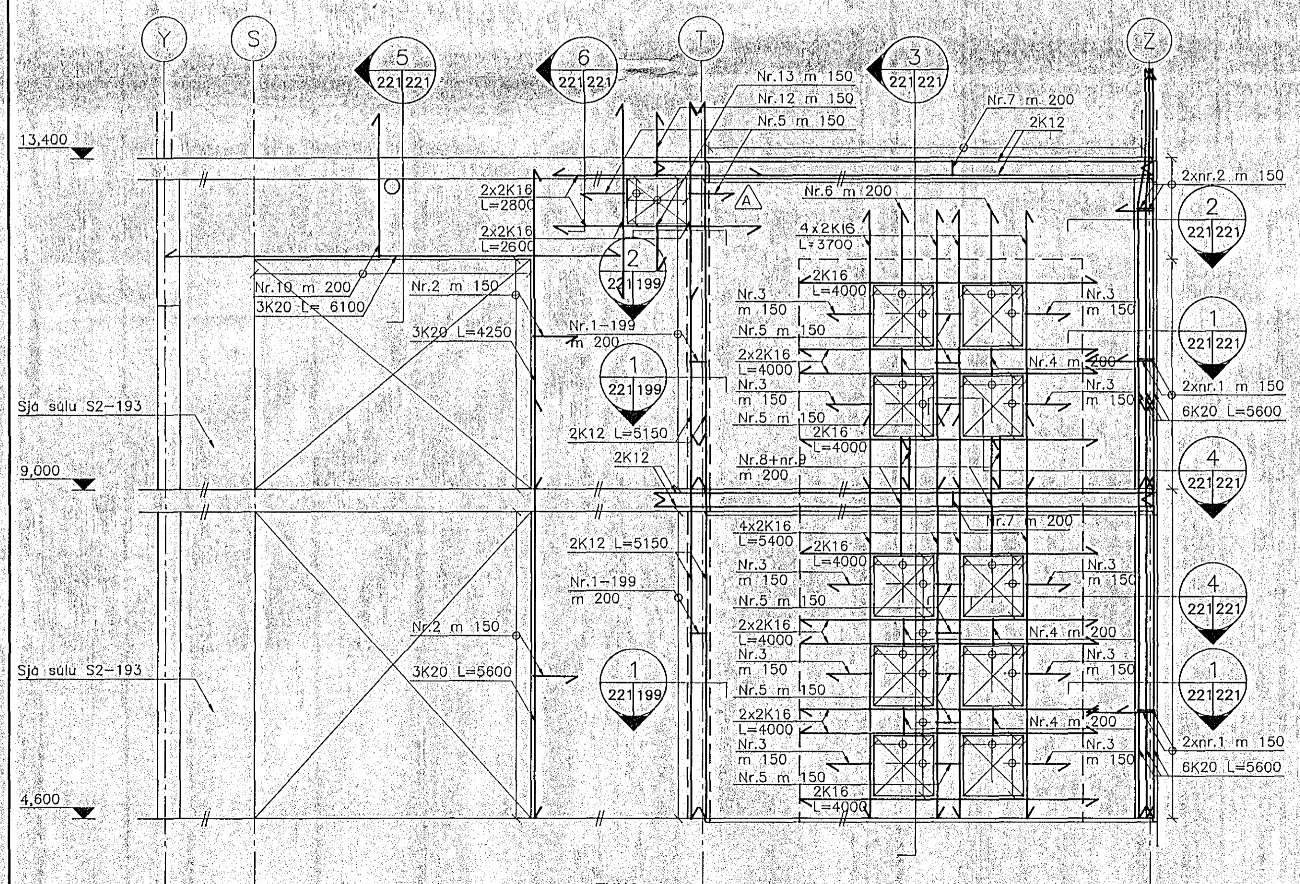
B HLIDARMYND 176/221 186 M 1:50
