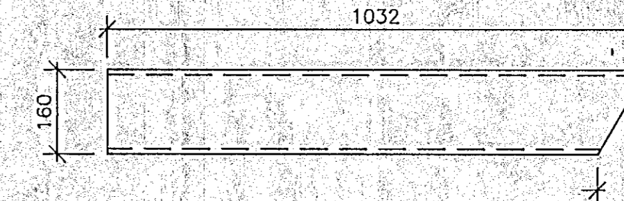
S28 U-160, L=1032, 1 stk. M. 1:10
