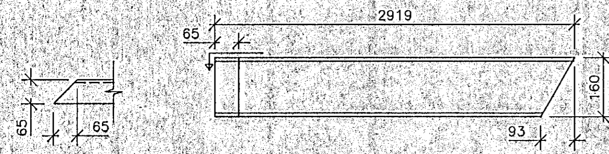
S5 U-160, L=2919, 1 stk. M. 1:10
