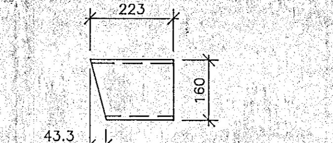
S30 U-160, L=223, 1 stk. M. 1:10
