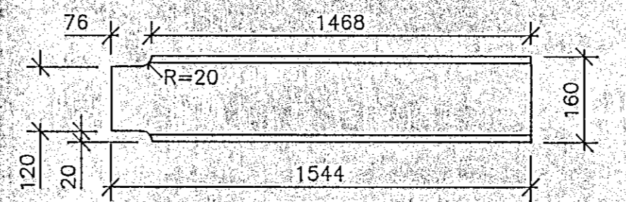
S25 HE160B, L=1544, 2 stk. M. 1:10
