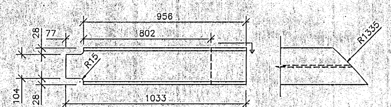
S13 HE160B, L=1033, 2 stk. M. 1:10
