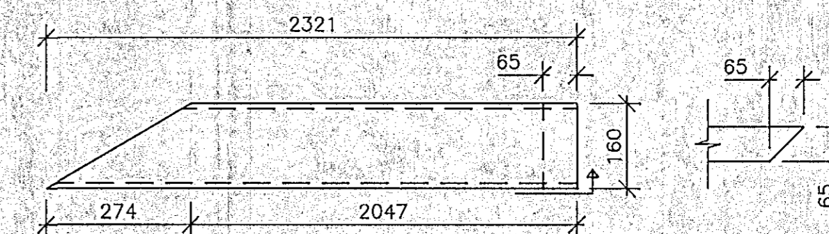
S27 U-160, L=2321, 1 stk. M. 1:10
