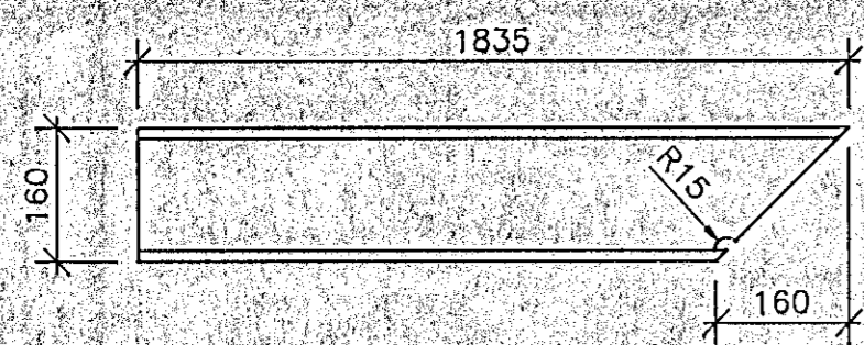
S8 HE160B, L=1835, 1 stk. M. 1:10
