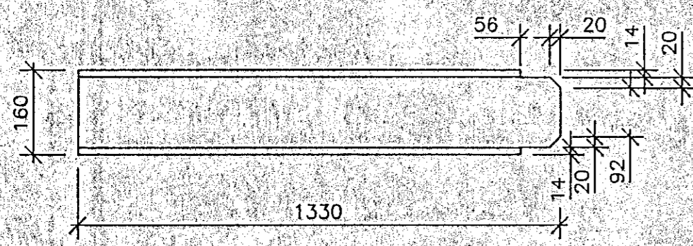
S7 HE160B, L=1330, 1 stk. M. 1:10
