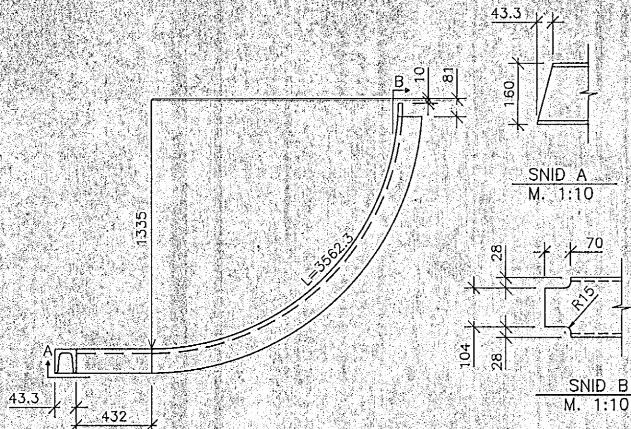
S11 U-160, L=3562.3, 1 stk. OKVARDAD
