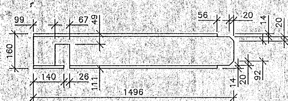
S6 HE160B, L=1496, 1 stk. M. 1:10
