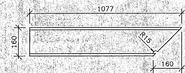
S9 HE160B, L=1077, 1 stk. M. 1:10
