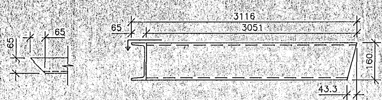
S4 U-160, L=3116, 1 stk. M. 1:10
