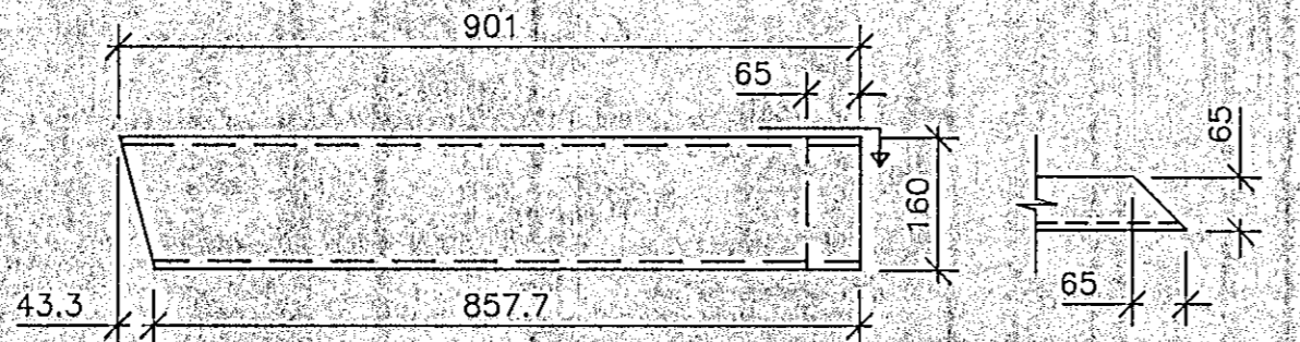
S16 U-160, L=901, 1 stk. M. 1:10
