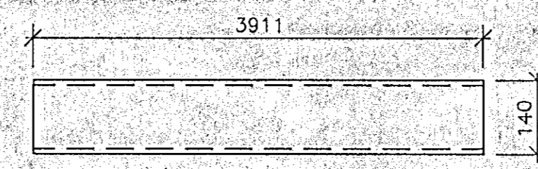
S22 U-140, L=3911, 1 stk. M. 1:10
