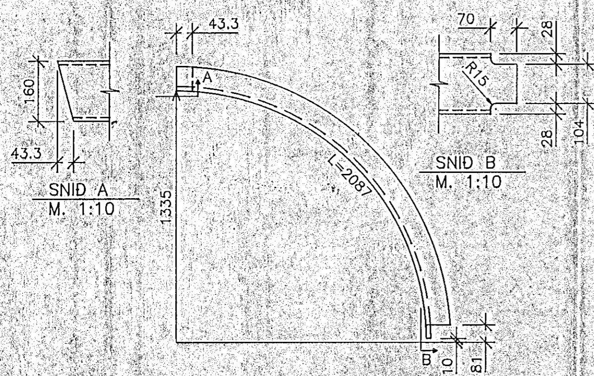
S10 U-160, L=2087, 1 stk. OKVARDAD
