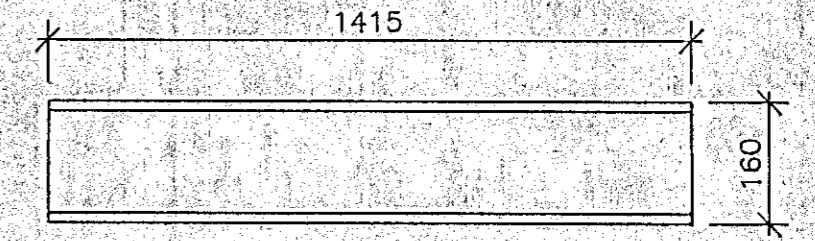
S31 U-160, L=1415, 1 stk. M. 1:10
