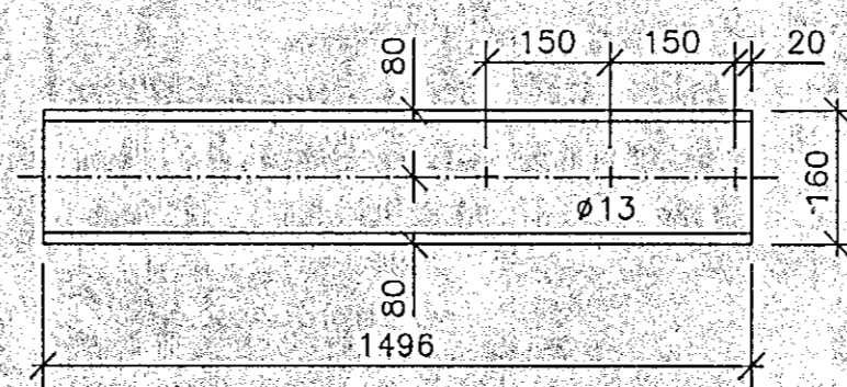
S23 U-160, L=1496, 1 stk. M. 1:10
