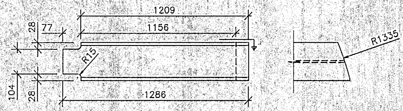
S12 HE160B, L=1286, 2 stk. M. 1:10
