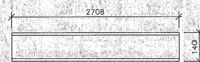
S18 U-140, L=2708, 1 stk. M. 1:10
