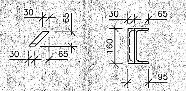
S15 U-160, L=95, 1 stk. M. 1:10
