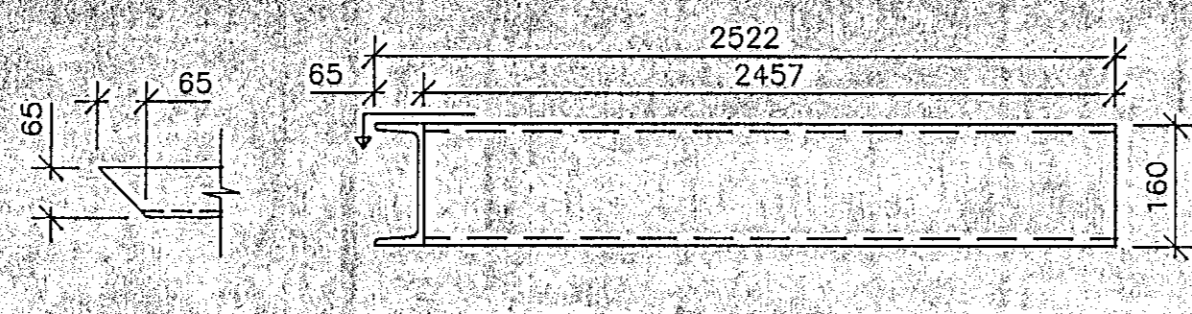
S14 U-160, L=2522, 1 stk. M. 1:10
