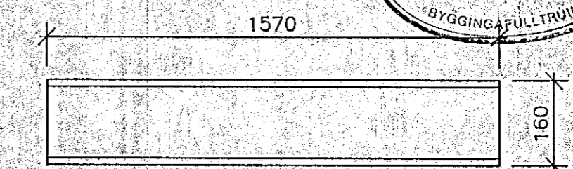
S33 U-160, L=1570, 1 stk. M. 1:10
