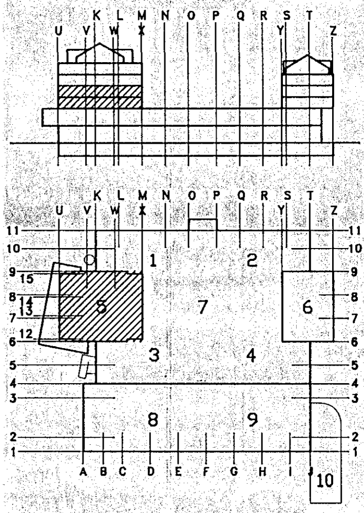
3 SNID 246/246 247 248 M. 1:20
