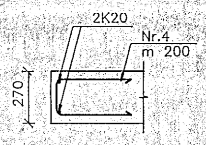
3 SNID 246/246 247 248 M. 1:20
