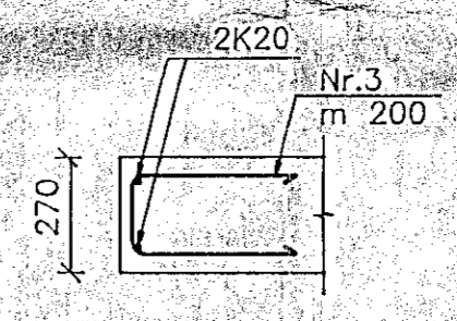
2 SNID 246/246 247 248 M. 1:20
