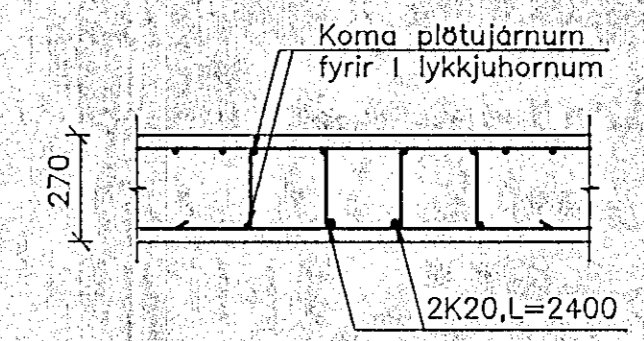
1 SNID 246/246 M. 1:20
