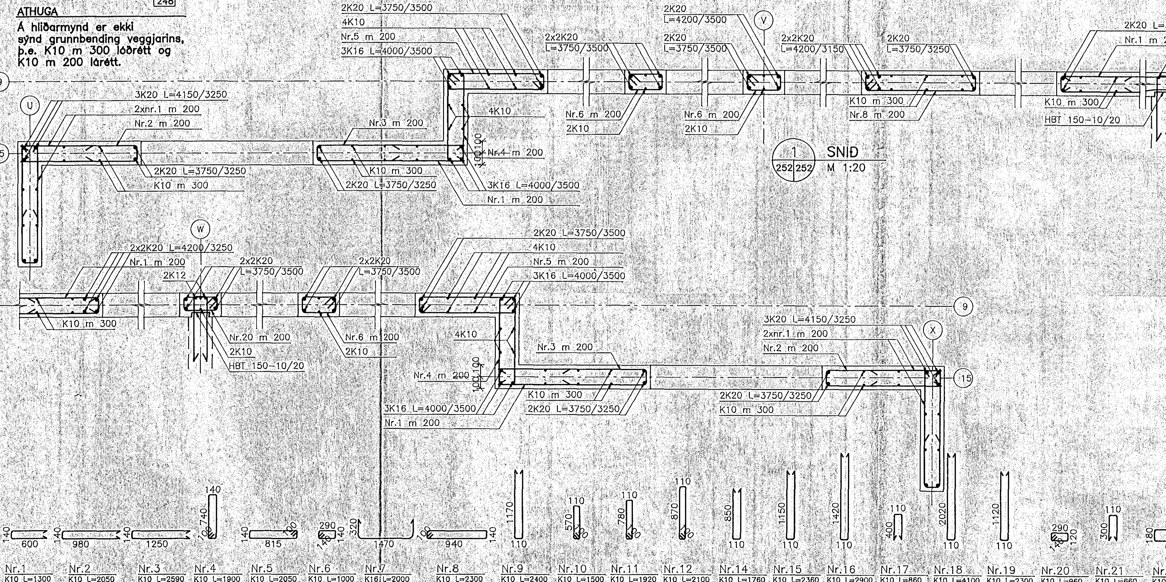
HLIDARMYND M 1:50
