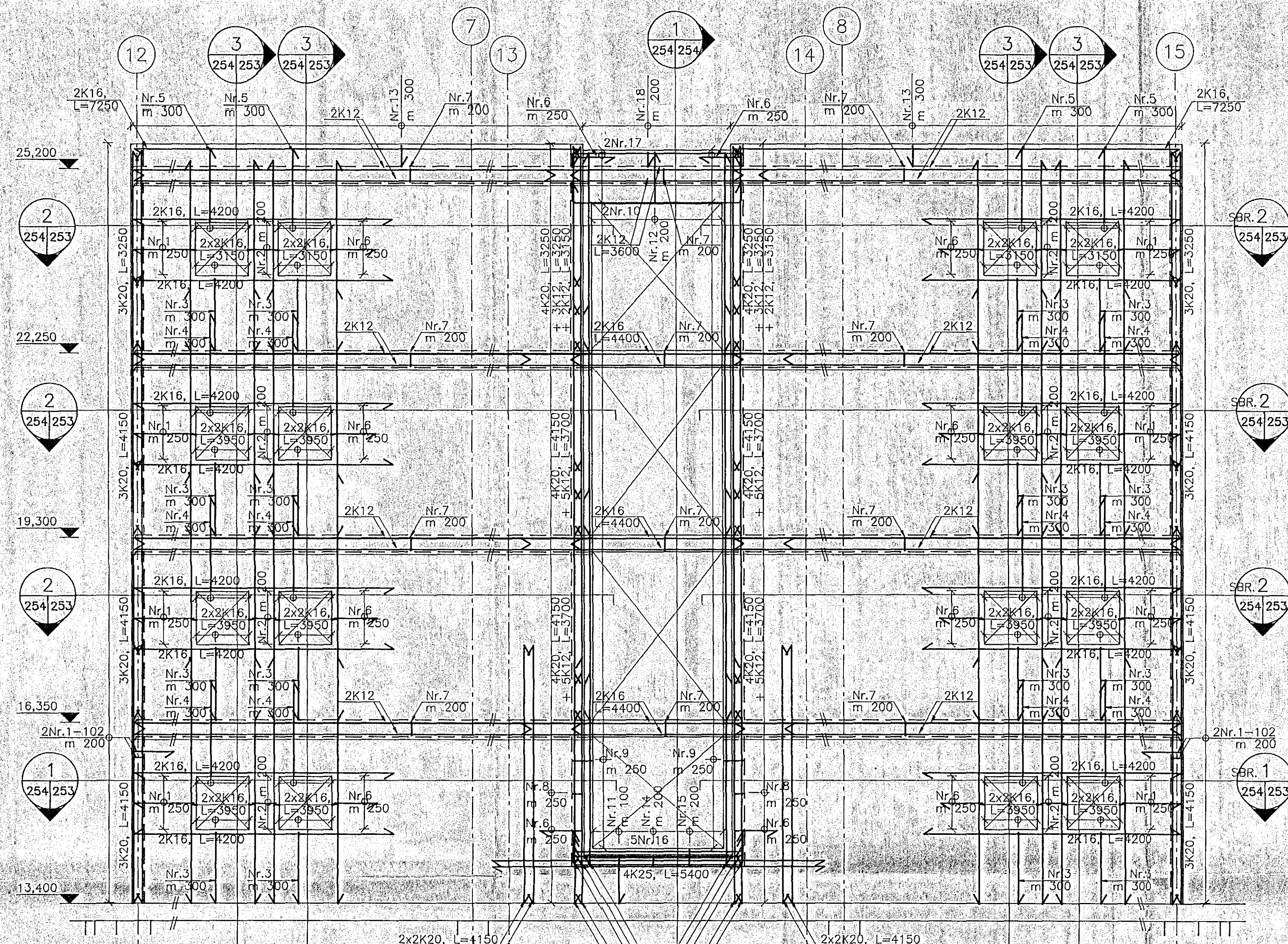
A HLIDARMYND M 1:50
