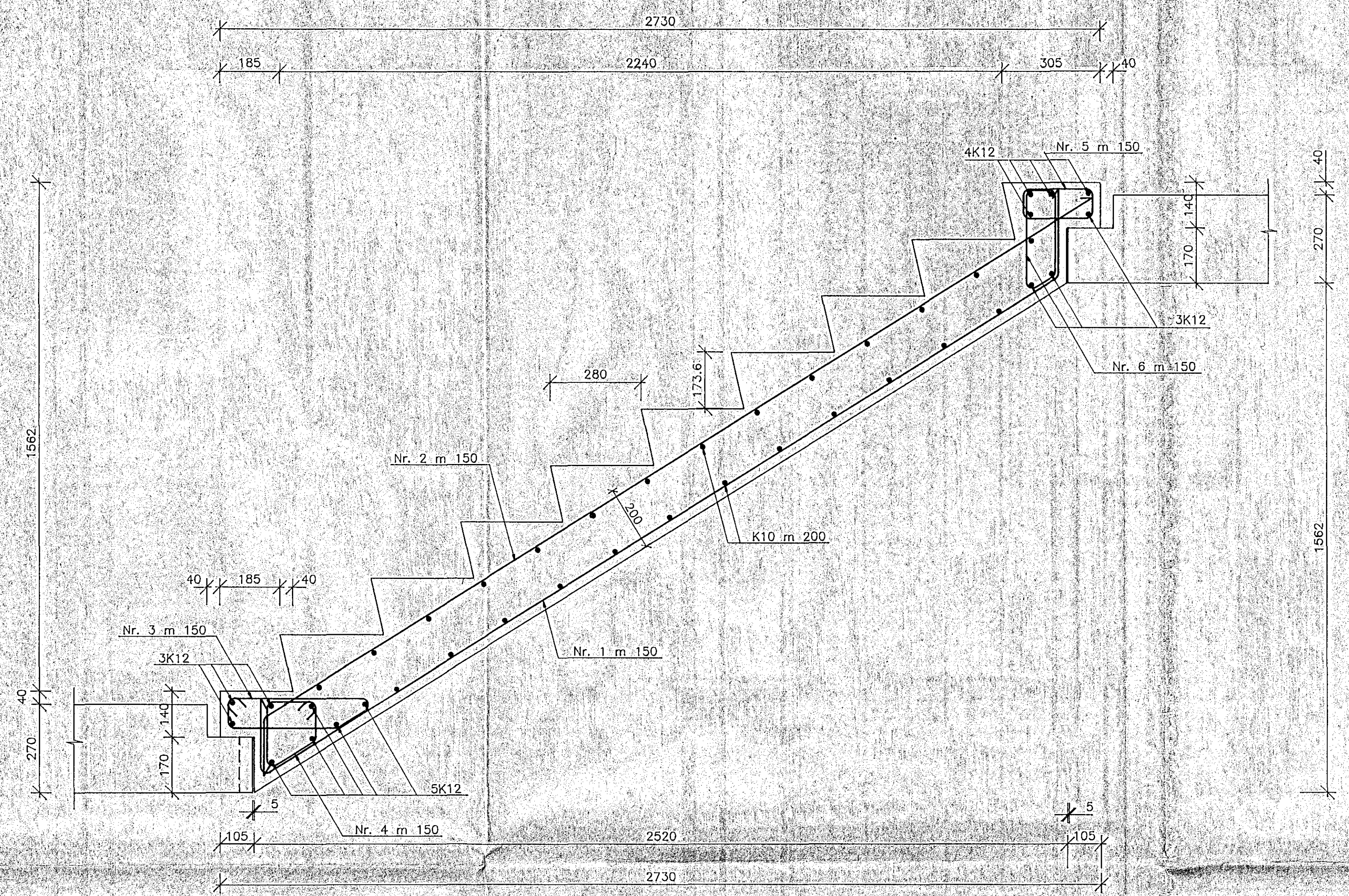
262/262 SNID I STIGAHLAUP MED 9 UPPSTIG, BREIDD=1400 ÖNNUR STIGAHLAUP SKULU JARNUD Á SAMA HÁTT M. 1:10
