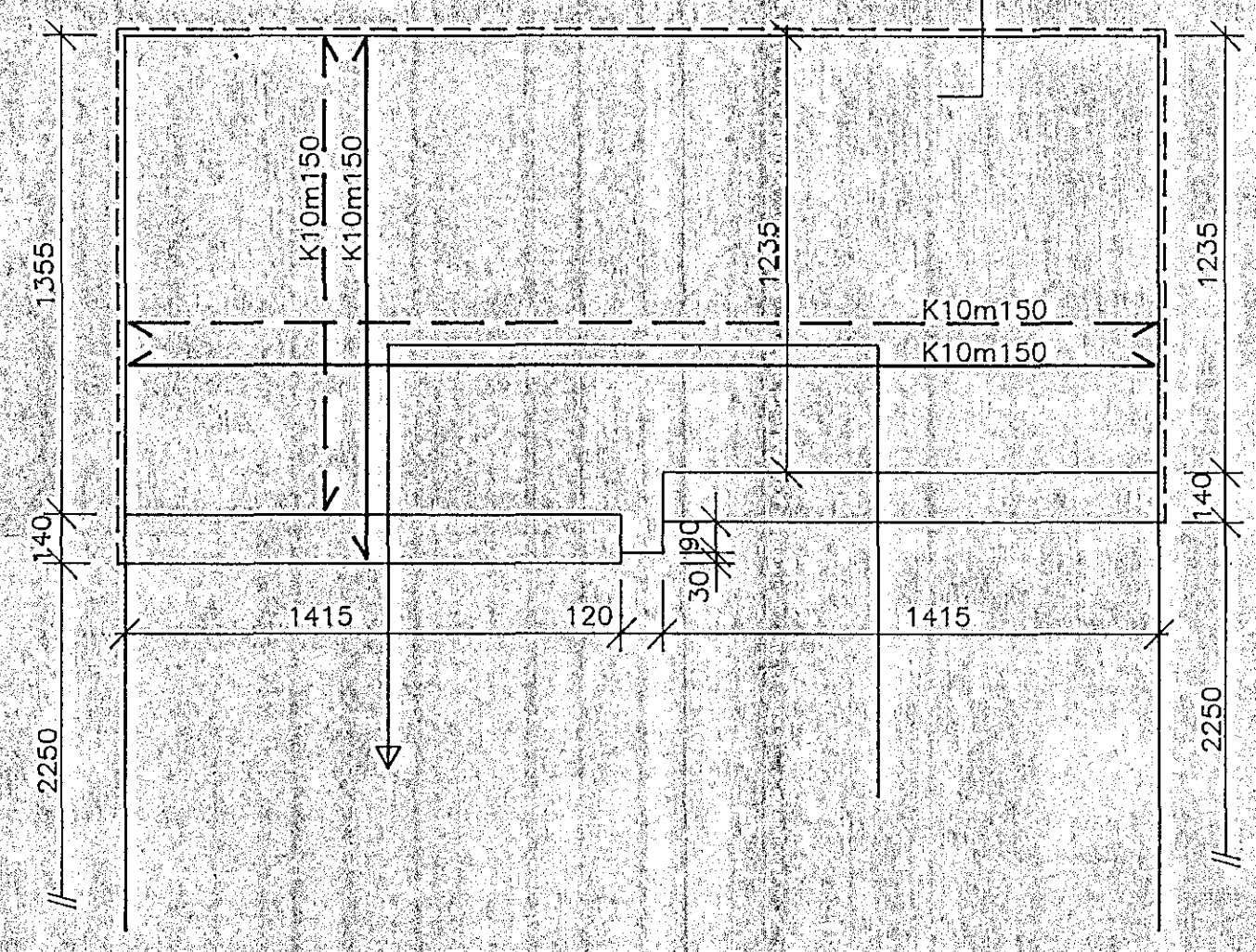
262/262 GRUNNMYND, STIGAPALLAR 3. TIL 6. HÆÐ M. 1:20
