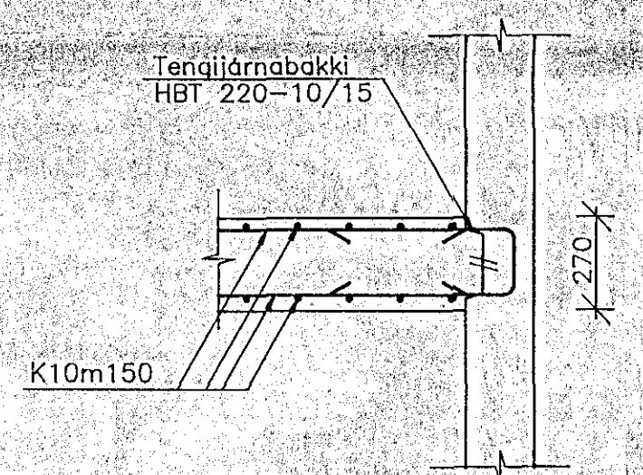
1 SNID 262/262 M. 1:20
