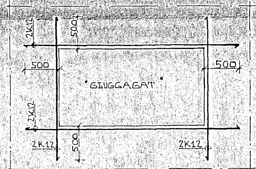
JARN KRINGUM GIUGGA EÐA DYR NEMA ANNAD SE SYNT A TEIKNINGUM
