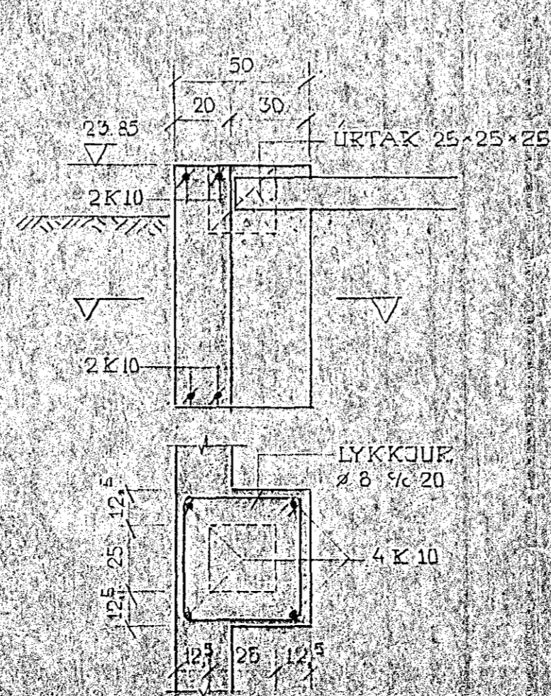
U3, 1:20
