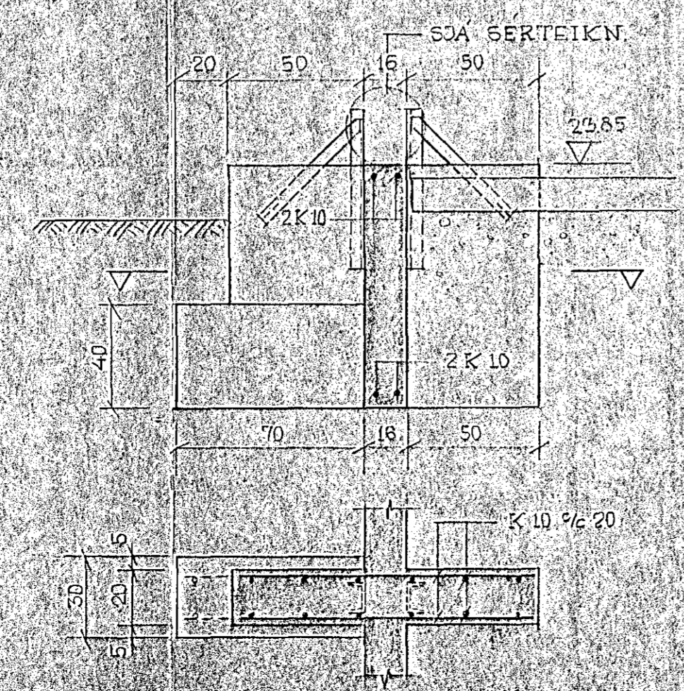
U2, 1:20
