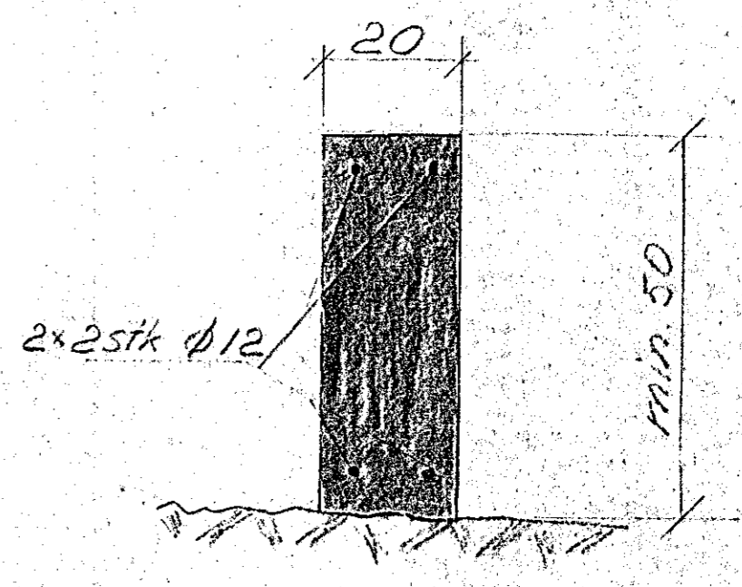
"A-A": Sneiðing í veggsockla. Mkv. 1:10
