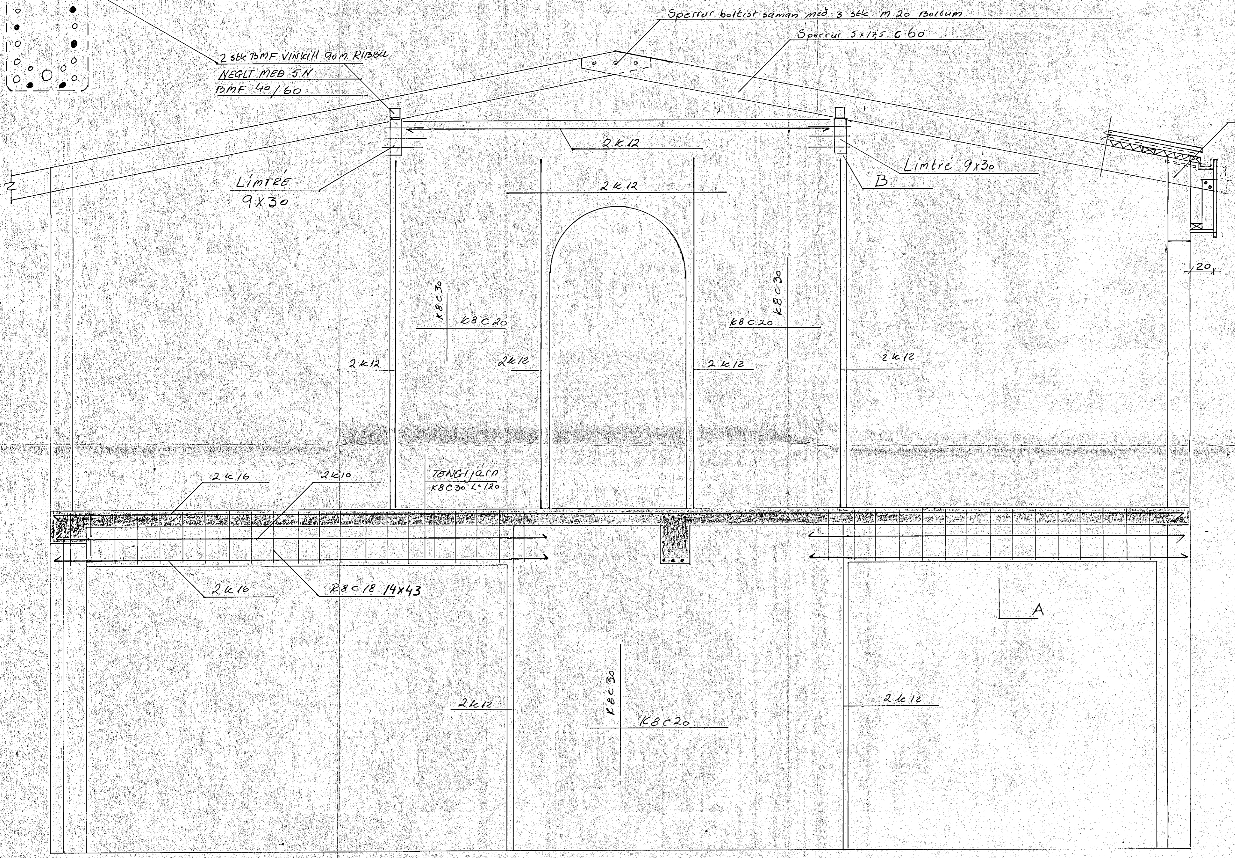
Steptur milliveggur 1:20
