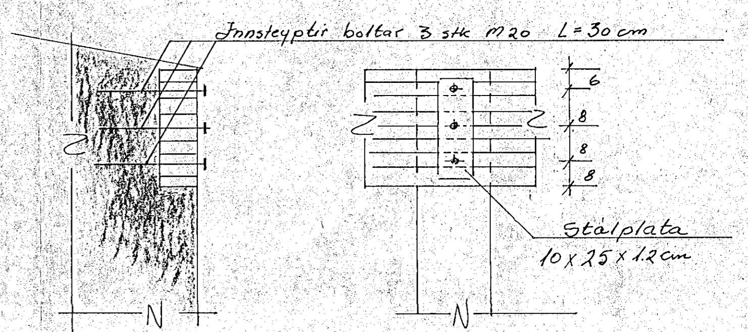
SÉRMYND B 1:10
