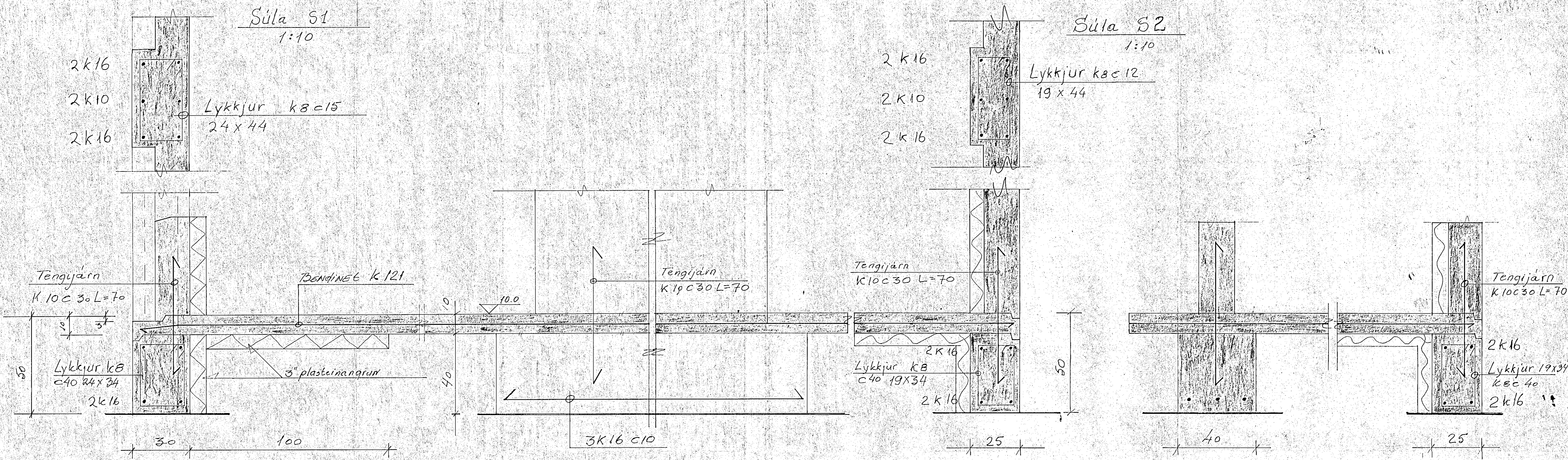
Snið B-B 1:10
