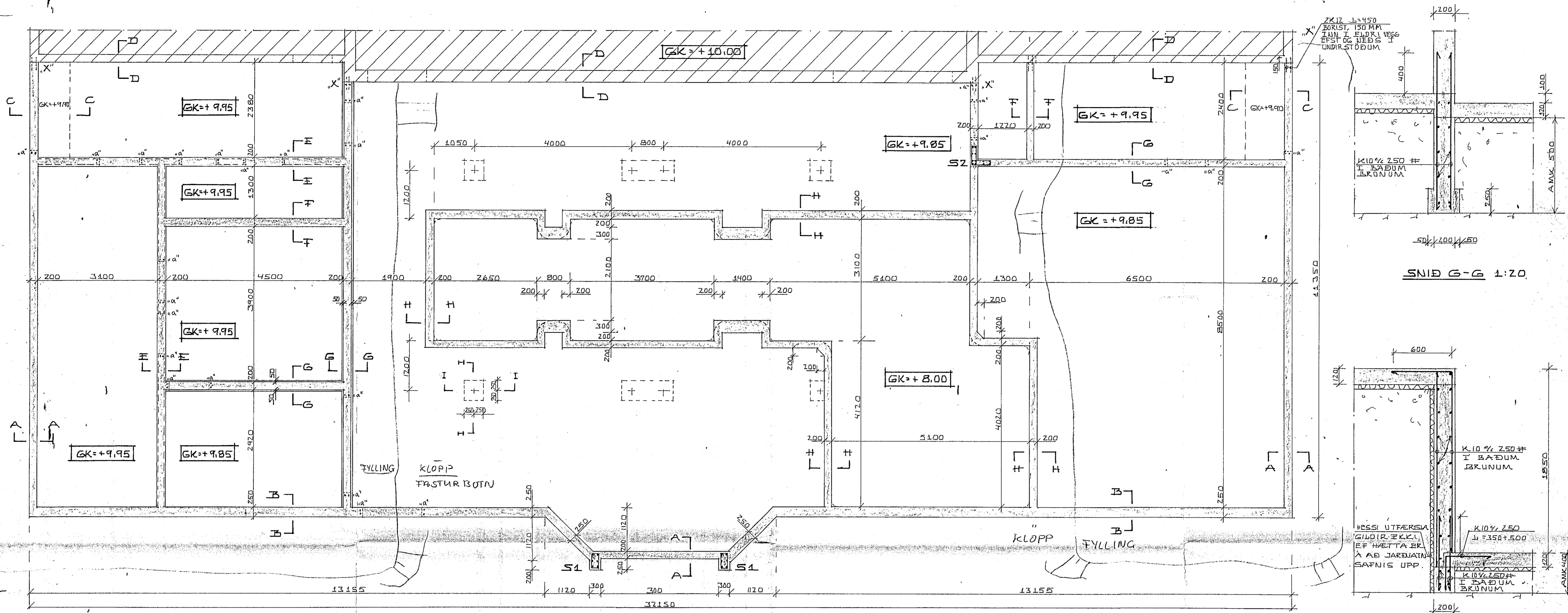
GRUNNMYND 1:50
