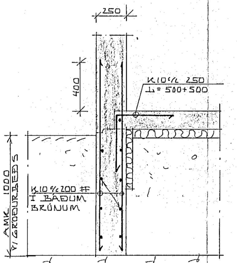
SNID B-B 1:20
