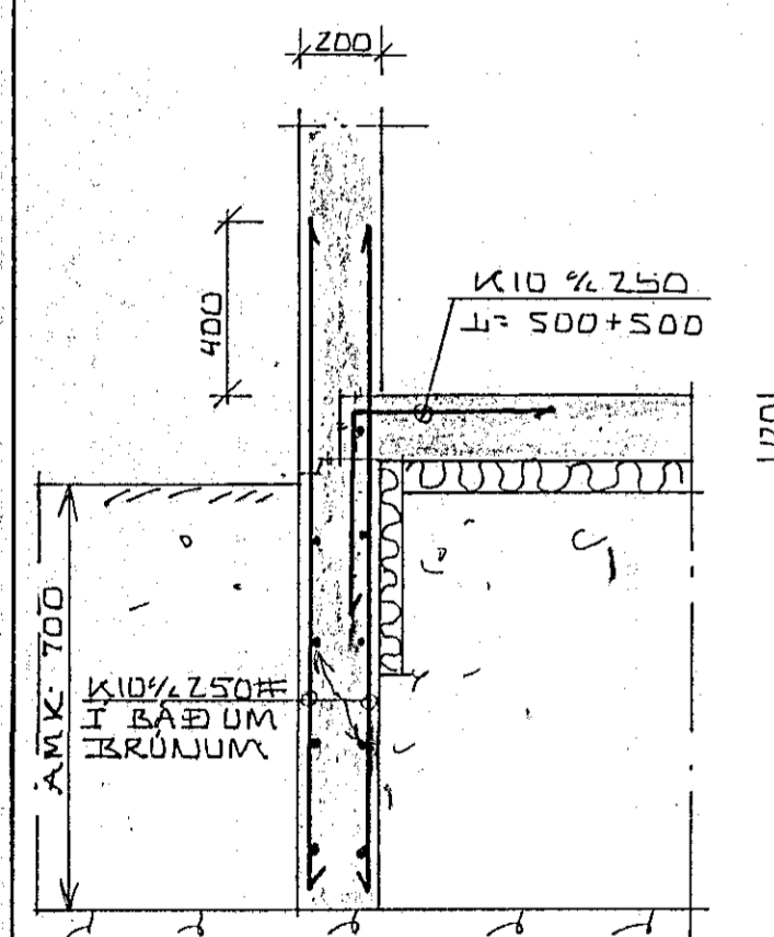
SNID A-A 1:20
