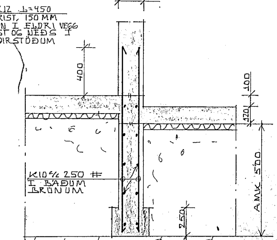
SNID G-G 1:20
