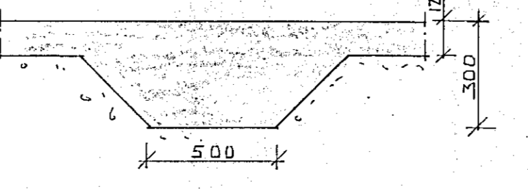
SNID I-I 1:20
