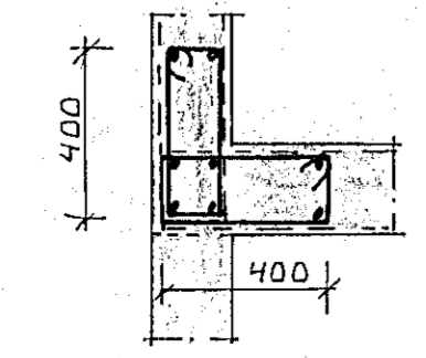
SNID I SÚLU S2 1:20
