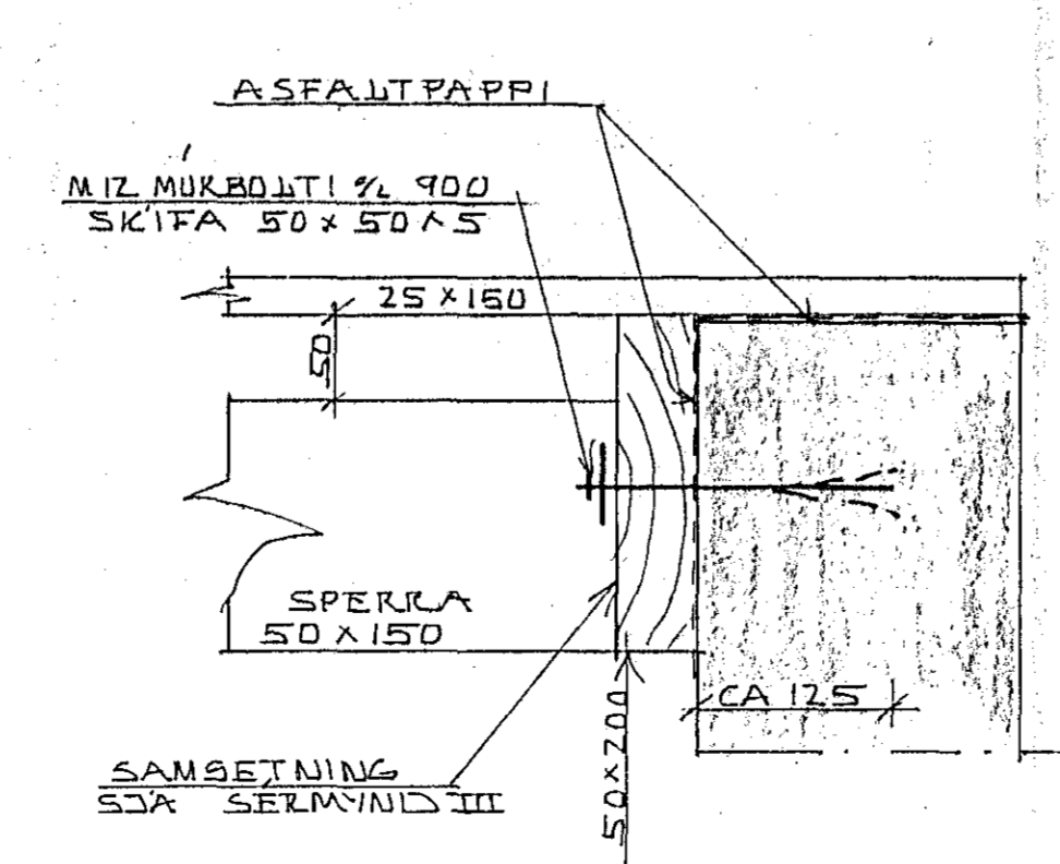
SNID D-D 1:5
