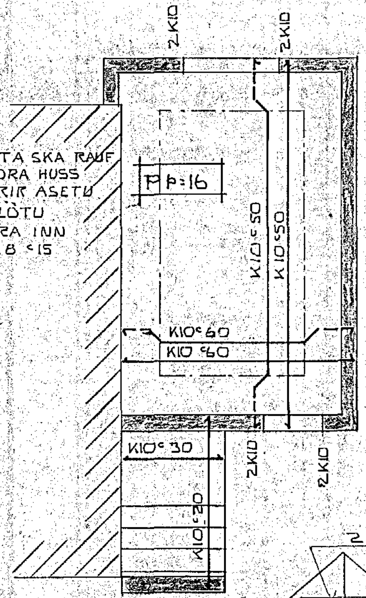
PLATA YFIR KJALLARA M 1:50
