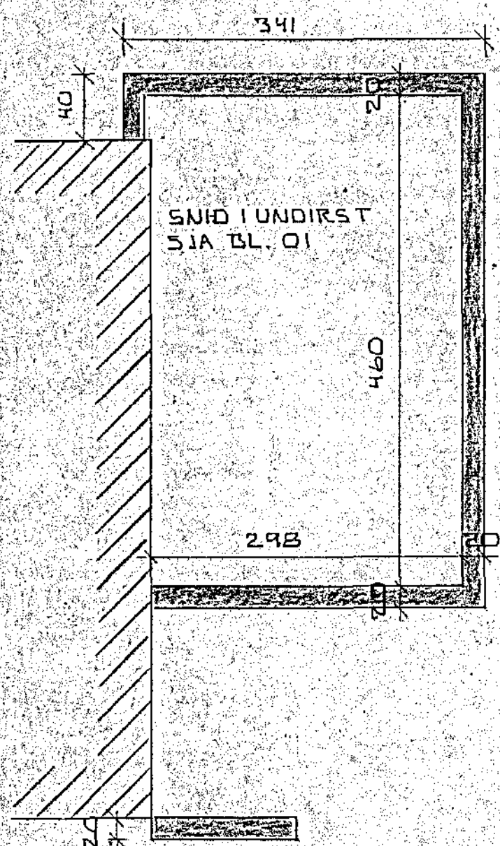
UNDIRSTÖÐUR M 1:50
