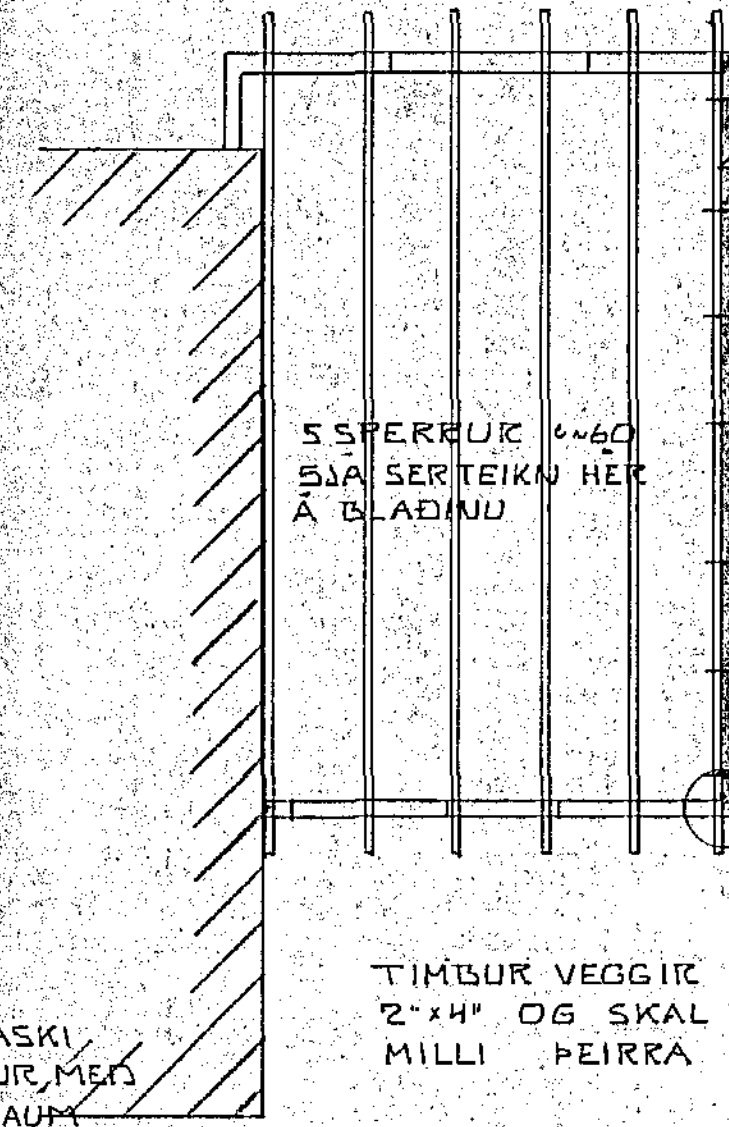
ÞAKVIÐIR M 1:50
