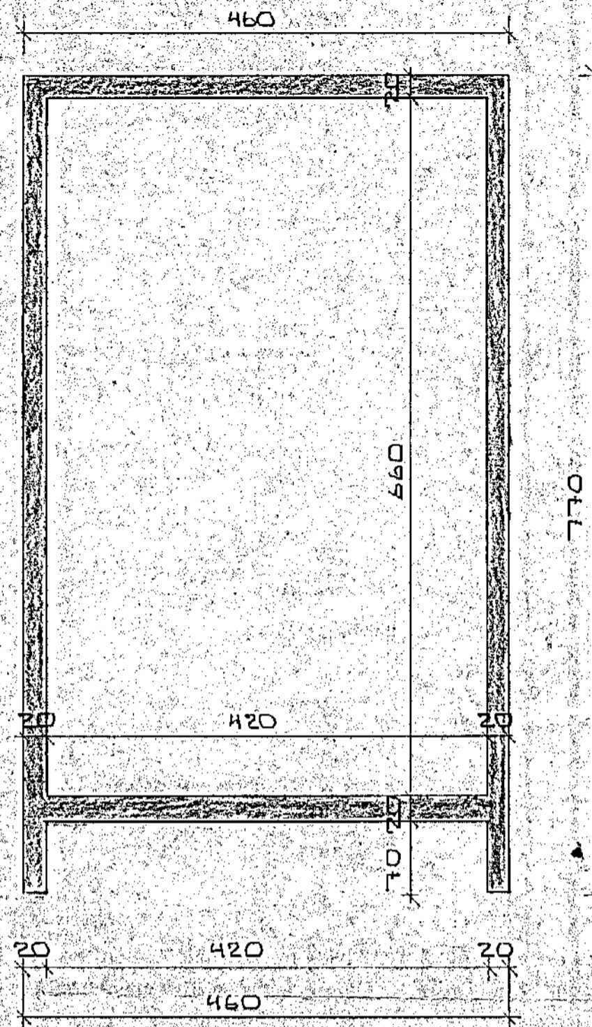
UNDIRSTÖÐUR M 1:50
