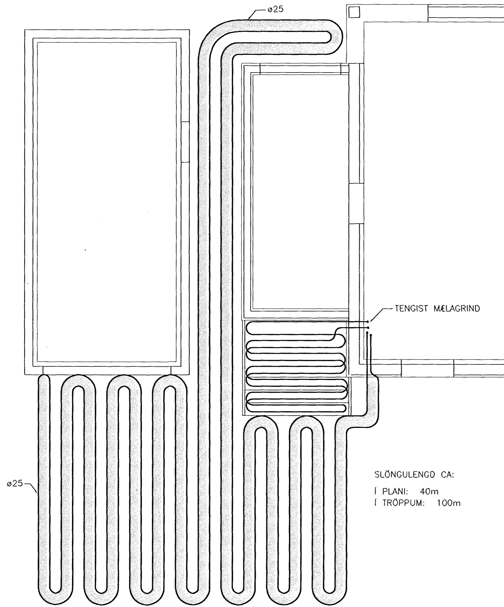
GRUNNMYND, 1:50
