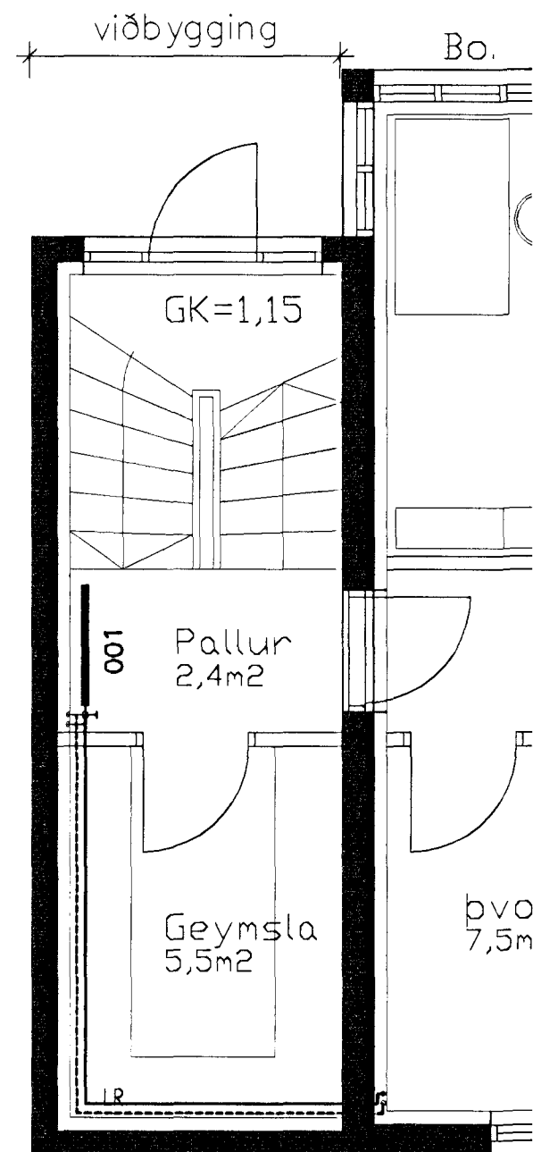
RIS GRUNNMYND, 1:50
