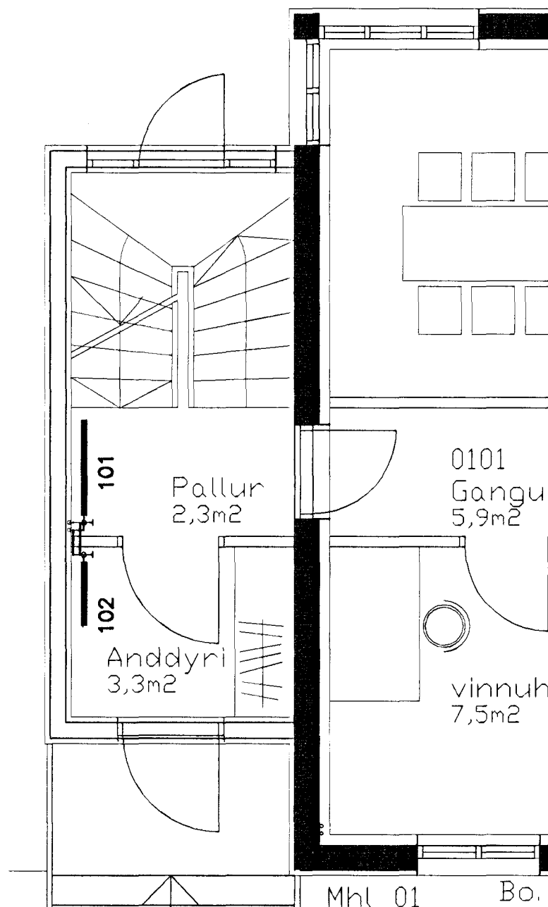
1 HÆÐ GRUNNMYND, 1:50
