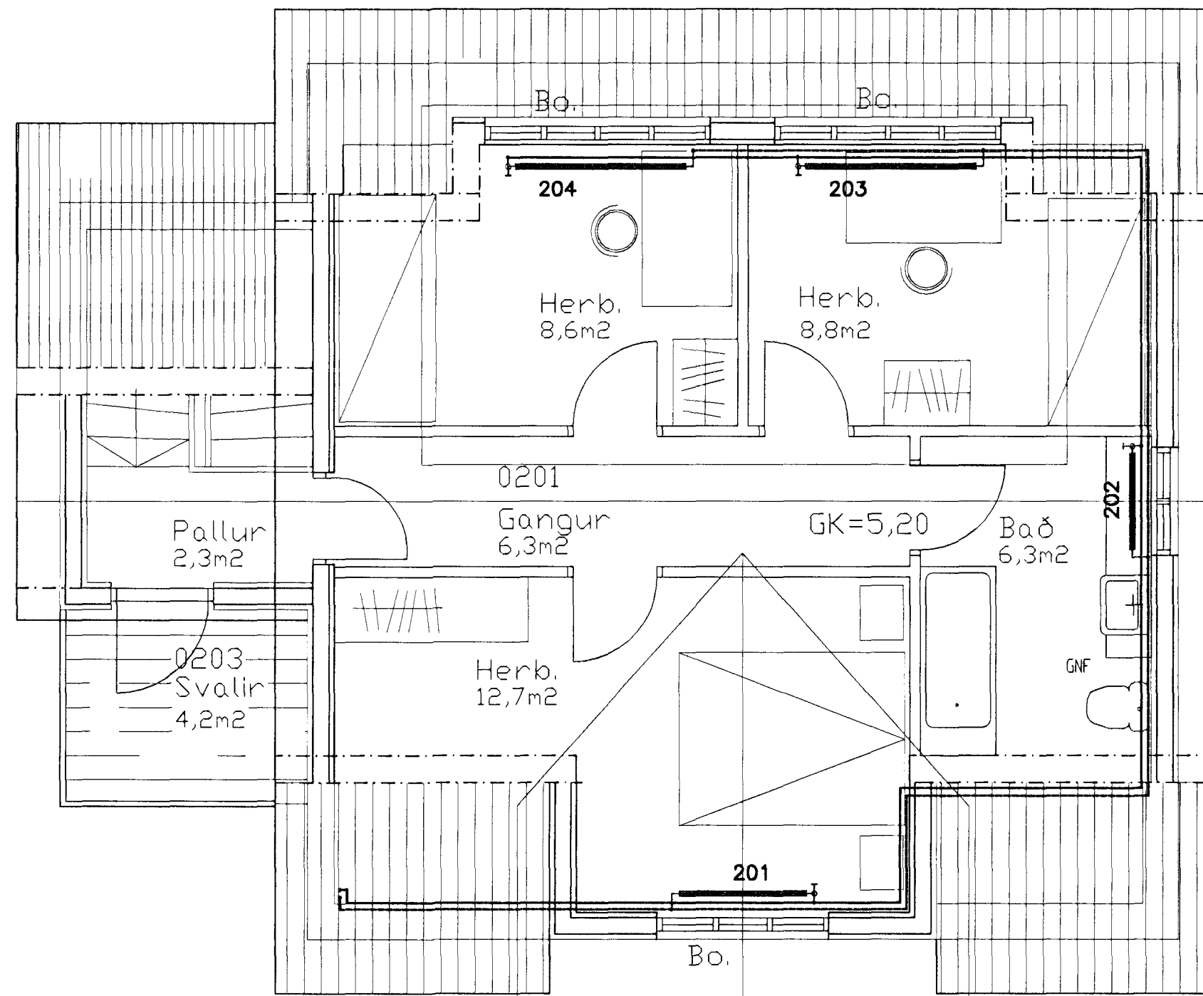
RIS GRUNNMYND, 1:50
