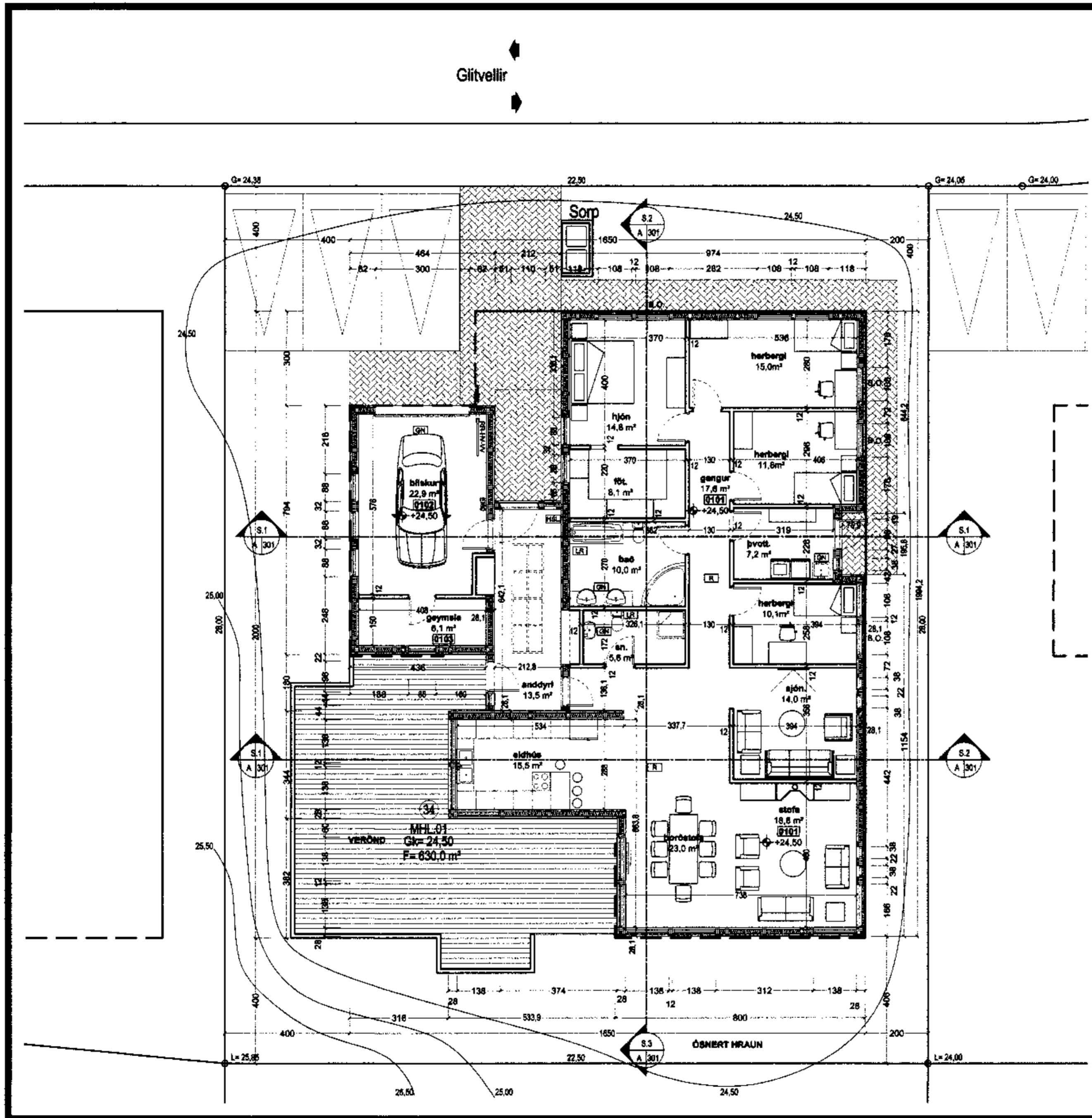
Grunnmynd 1:100
