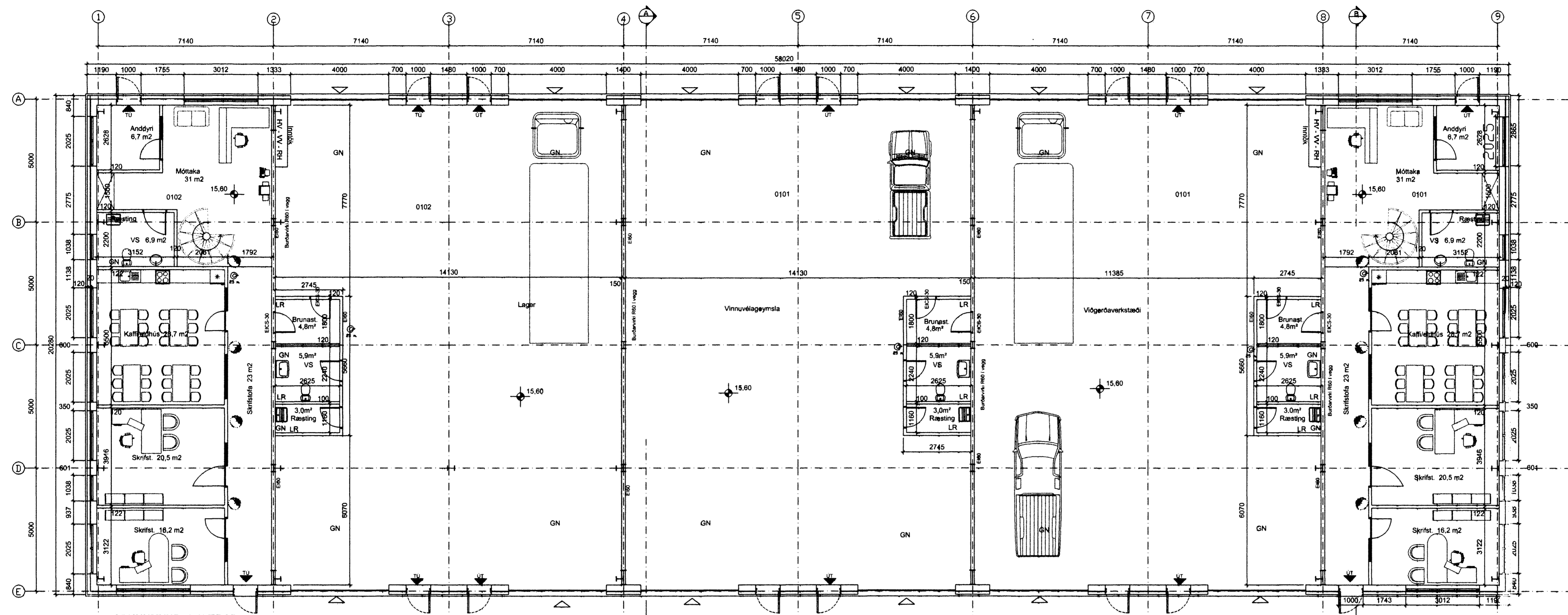
GRUNNMYND 1. HÆÐAR mhl. 01
