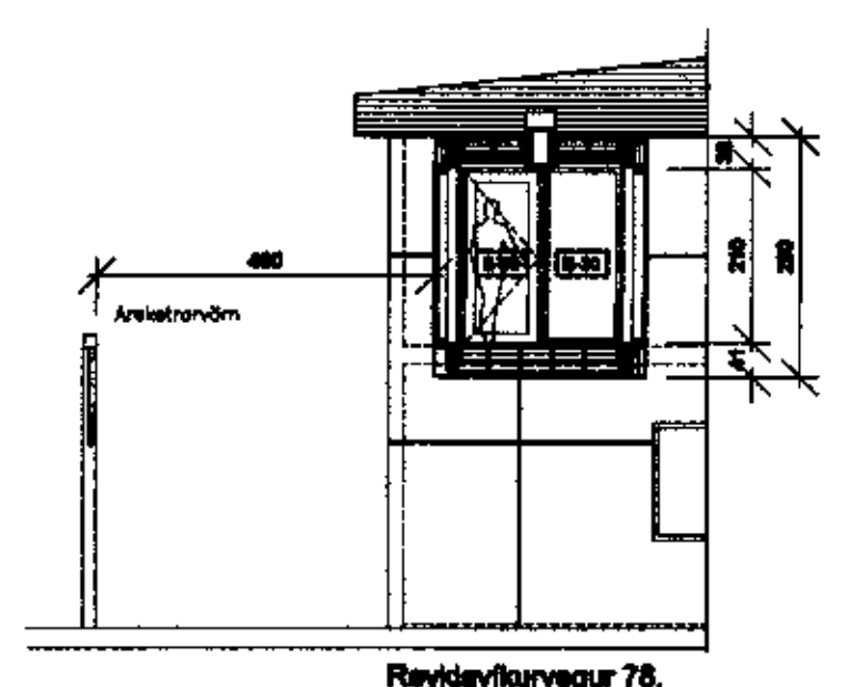
SNEIDING B-B 1:100
