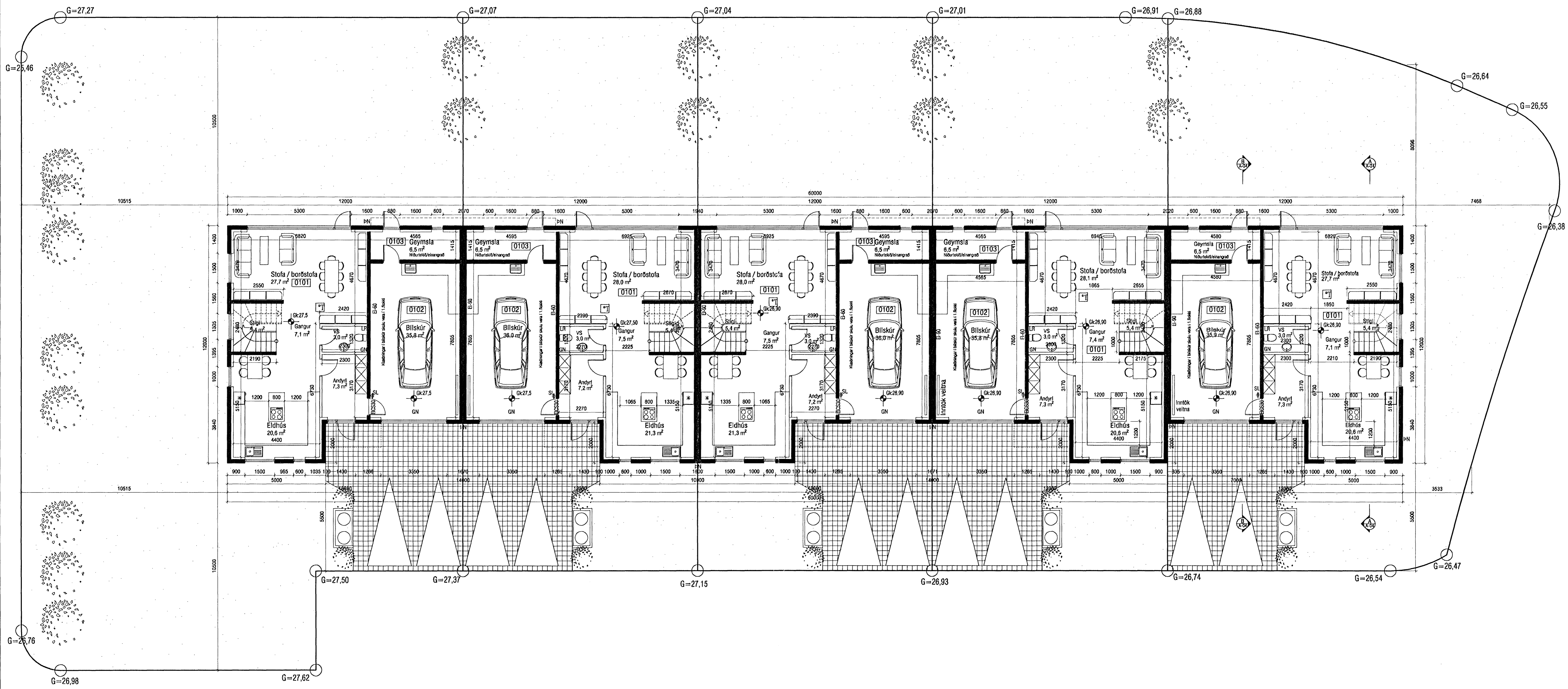
GRUNNMYND 1.HÆÐ 1:100
