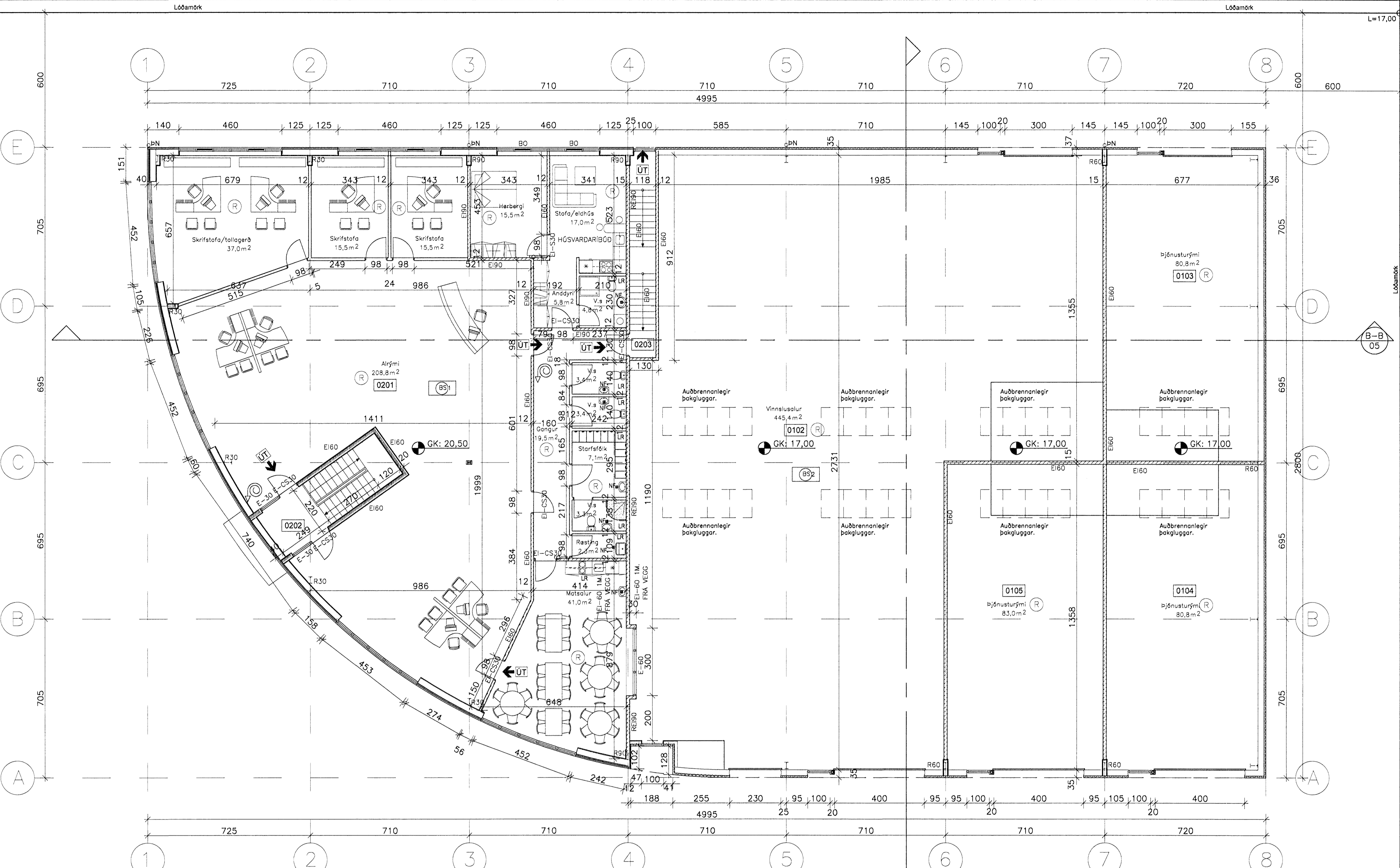
GRUNNMYND 2. HÆÐAR 1:100
