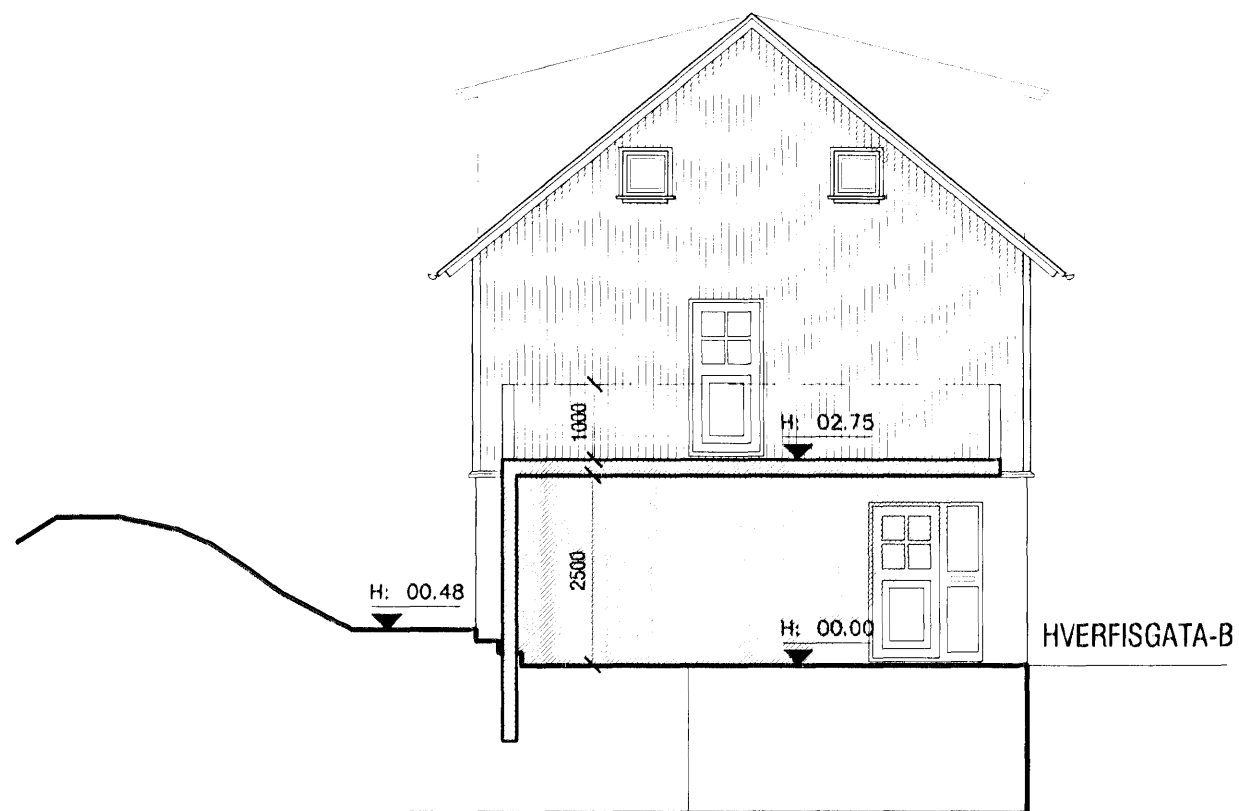
Ásýnd Norð-Austur mkv. 1:100
