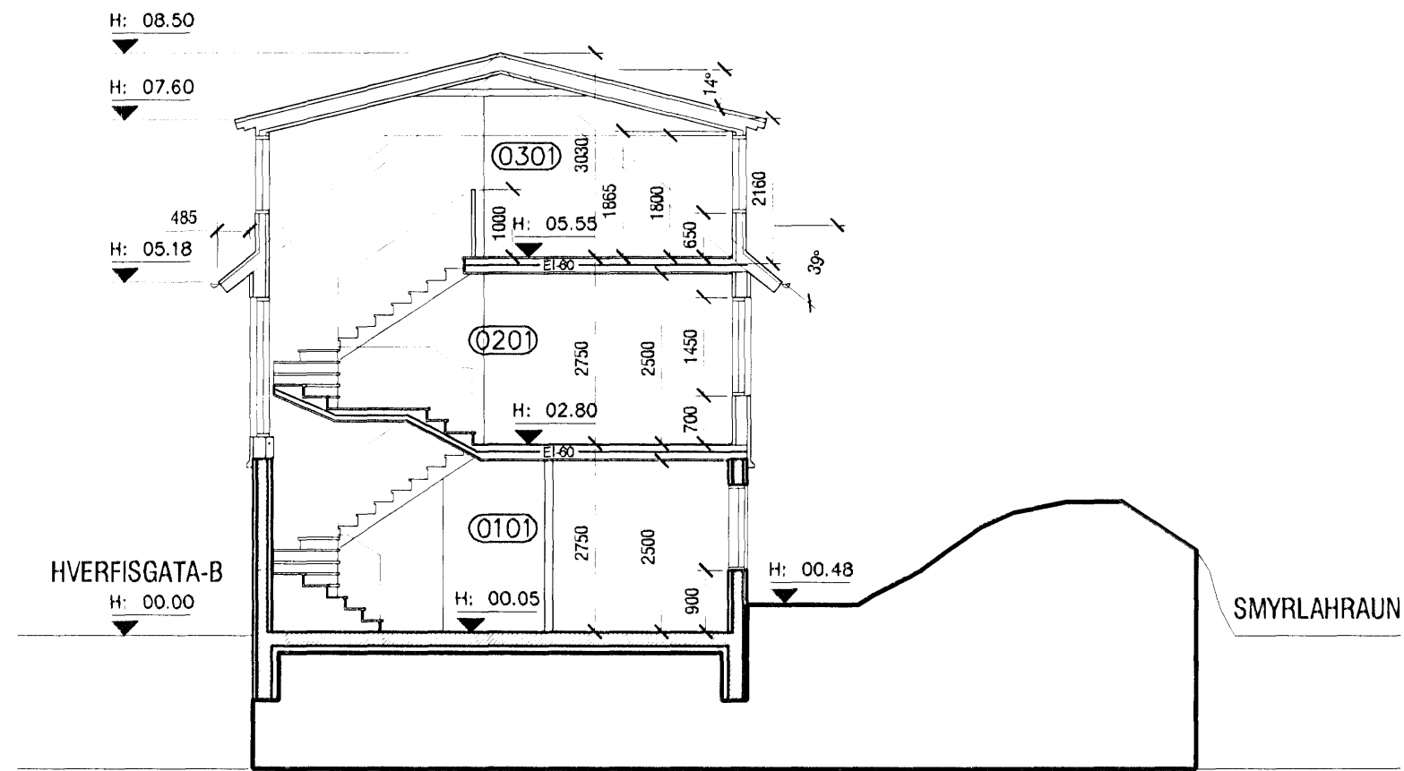
Sneiðing A-A mkv. 1:100
