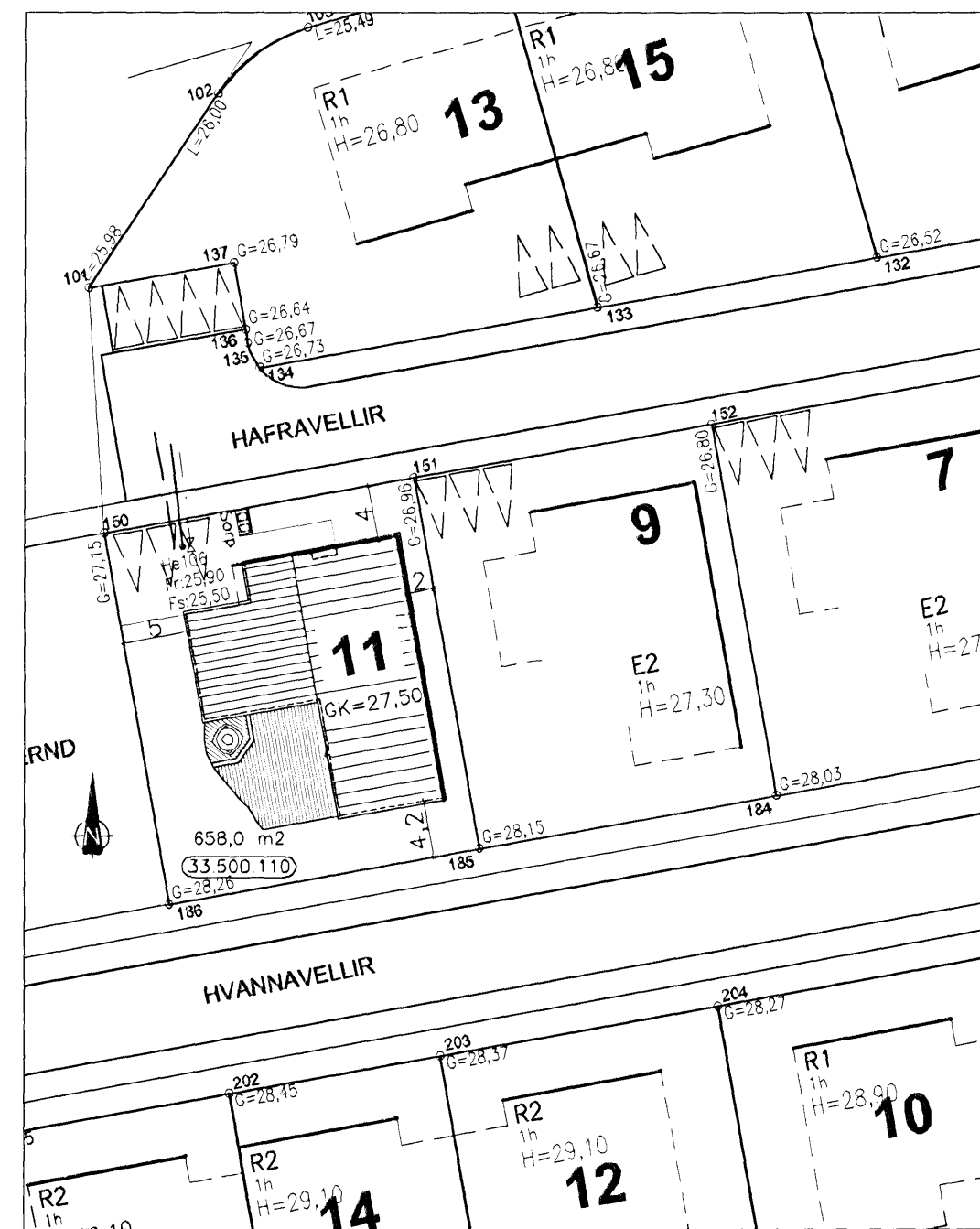
AFSTÖÐUMYND 1:500
