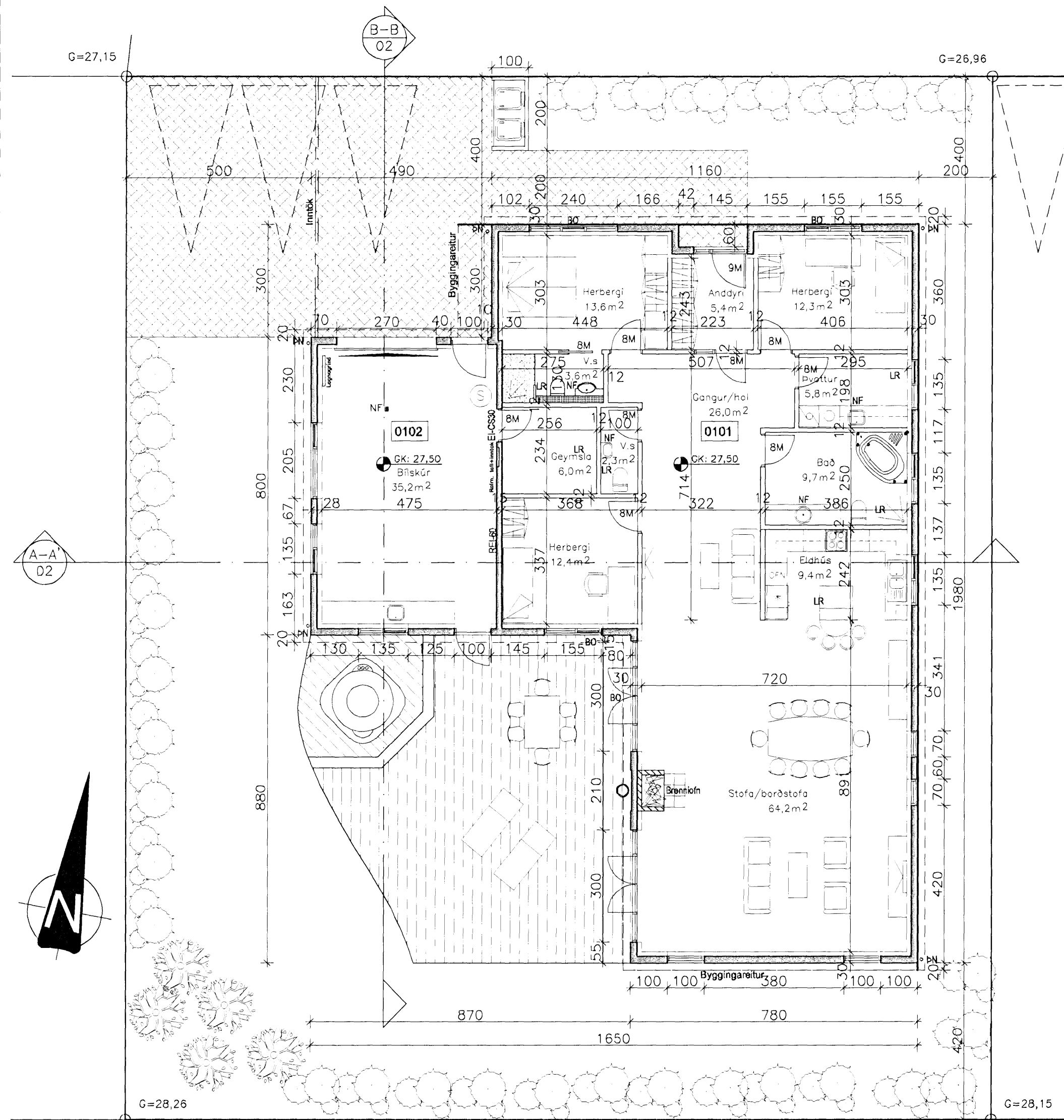
GRUNNMYND 1. HÆÐAR 1:100
