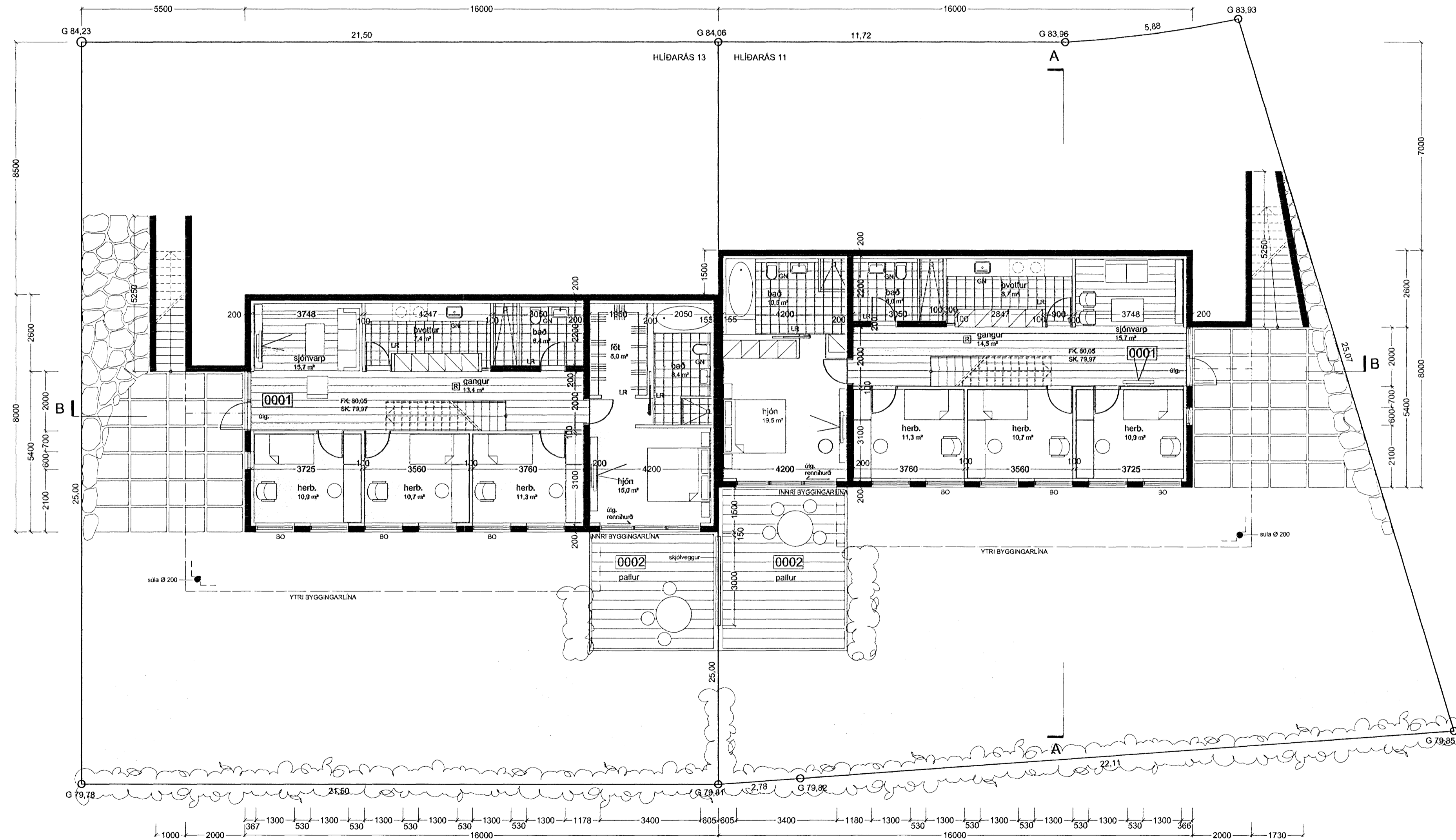
GRUNNMYND NEDRI HÆÐ M 1:100
