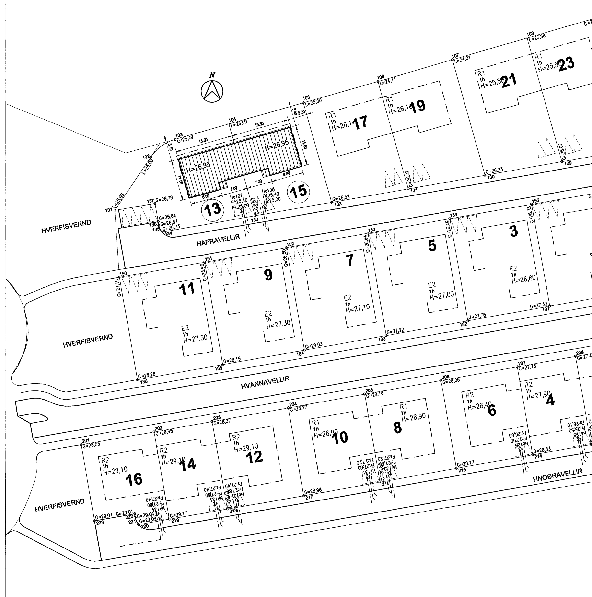
AFSTÖÐUMYND MKV. 1:500
