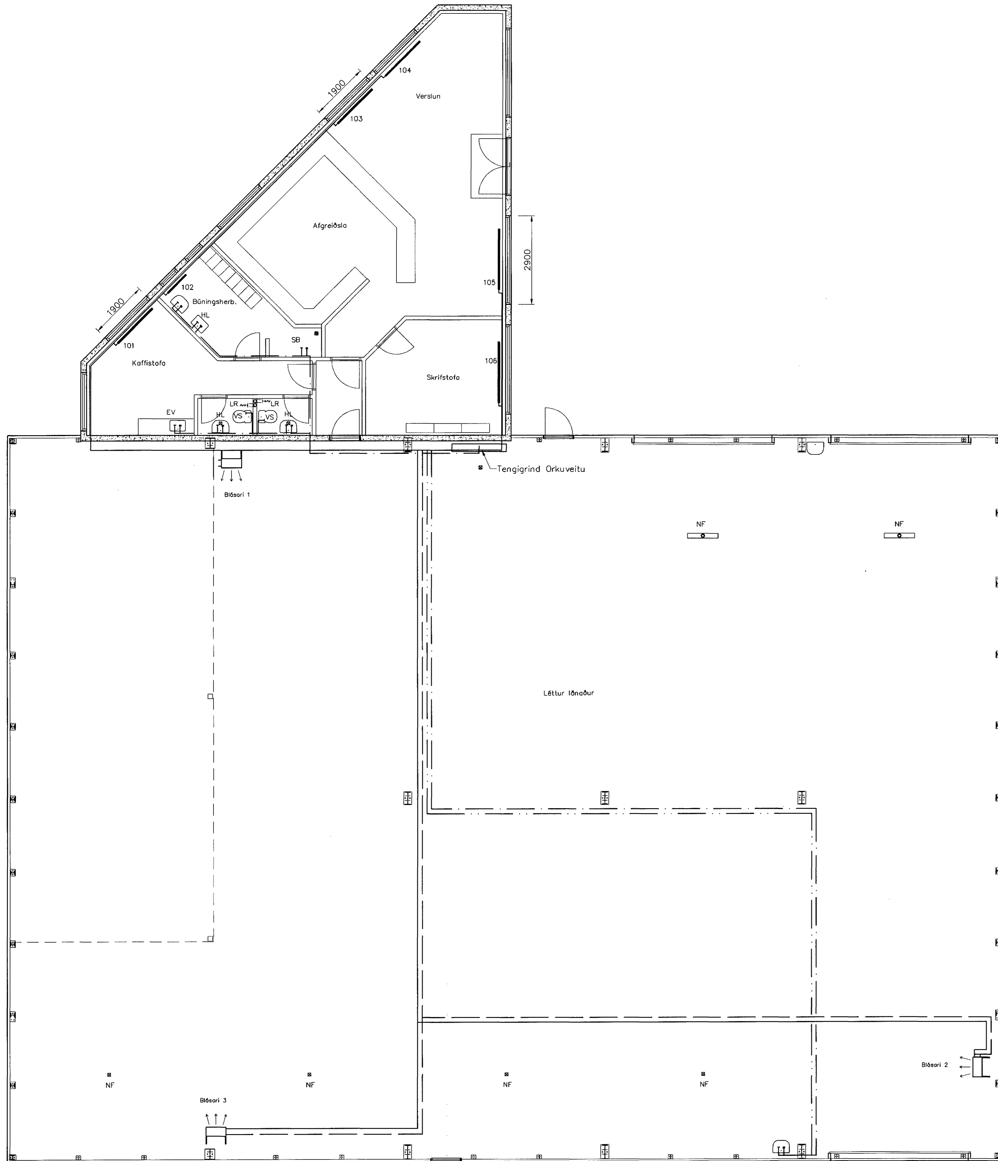
Lagnir, Grunnlag, 1:75
