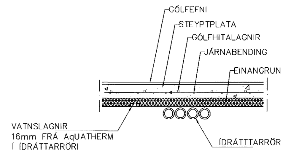
LAGNIR, SNIÐ, 1:20
