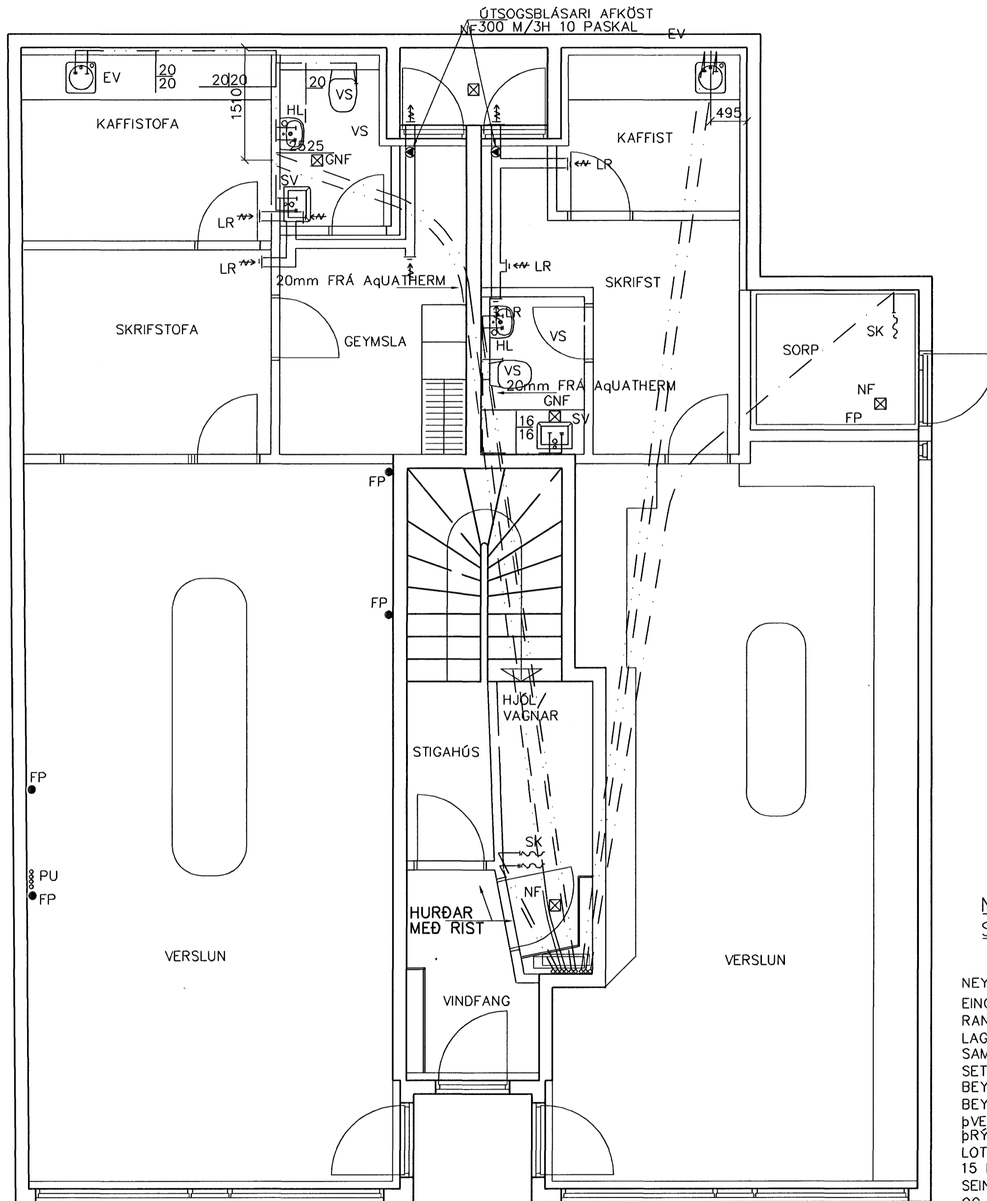
GRUNNMYND 1:50
