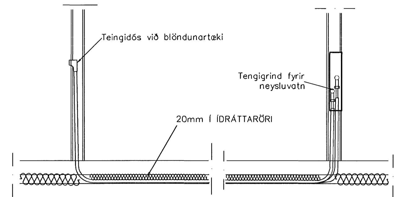
TENING NEYSLUVATNSLAGNA 1:20
