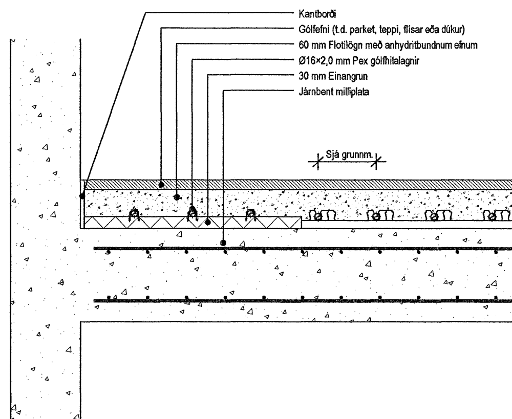
KENNISNIÐ GÓLFHITA 1:10
