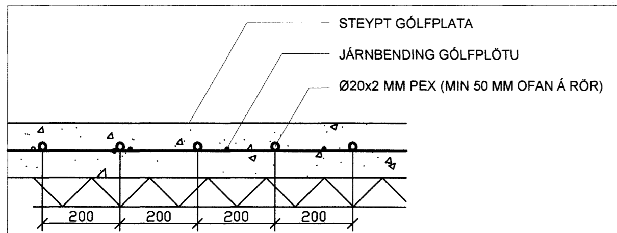
SNÍÐ Í GÓLFHITALÖGN - 1:10
