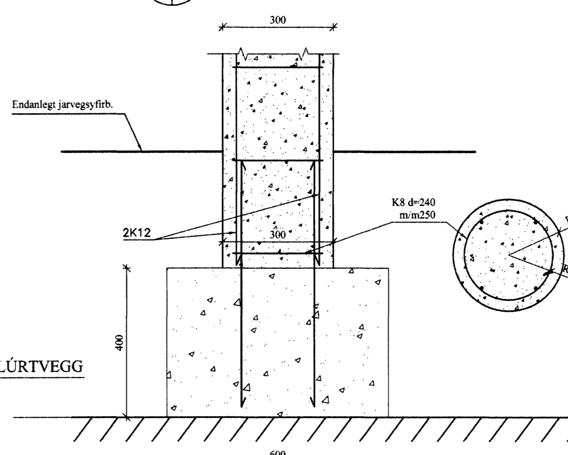
003 SKURÐUR Í SÖKKULÚRTVEGG Mkv: 1/10
