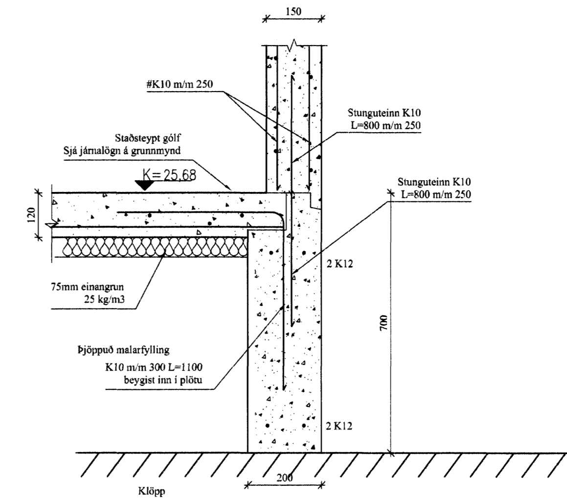
001 SKURÐUR Í SÖKKULÚRTVEGG Mkv: 1/10
