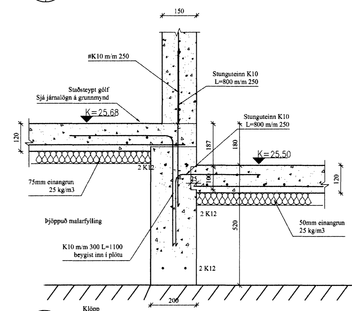
002 SKURÐUR Í SÖKKULÚRTVEGG Mkv: 1/10
