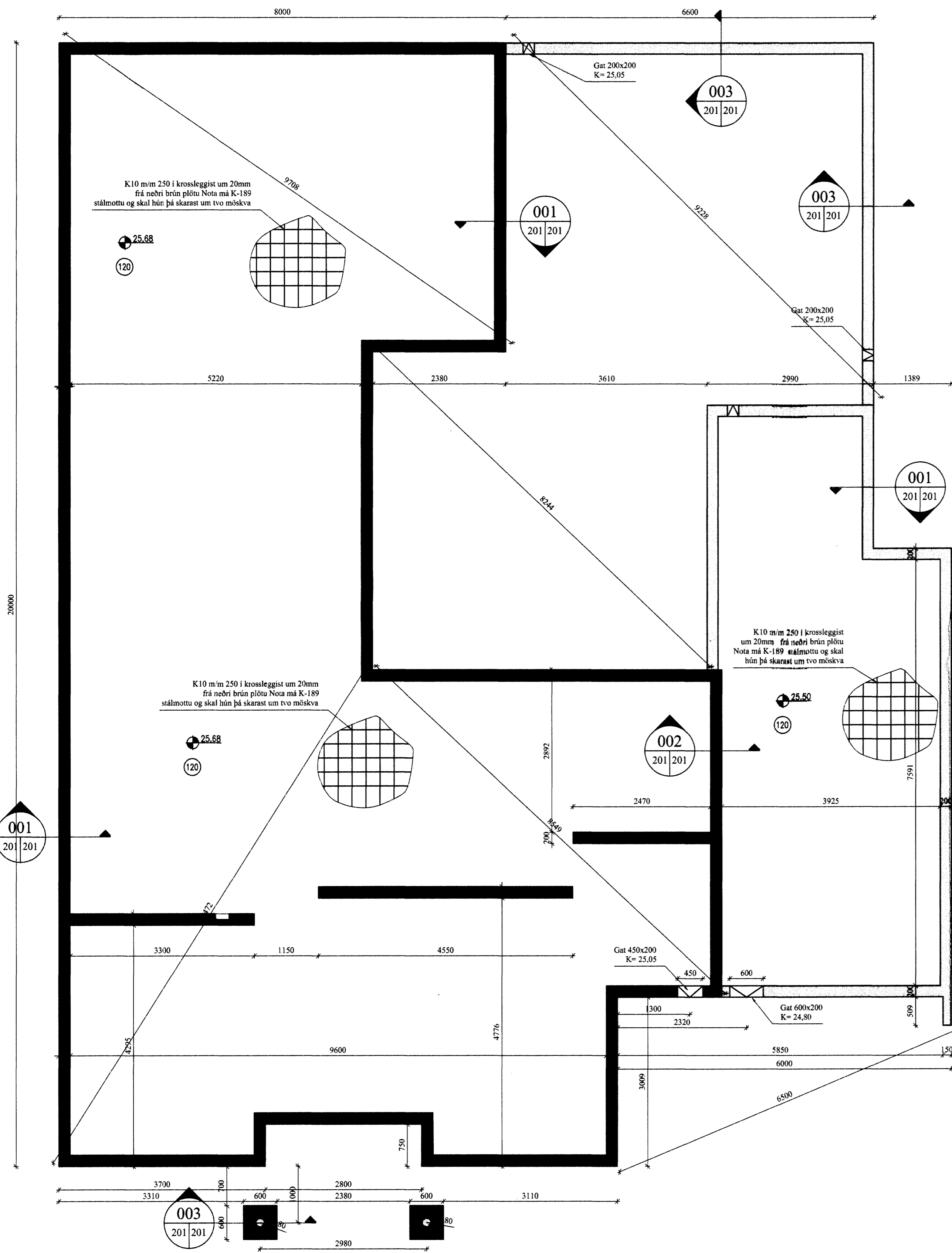
GRUNNMYND SÖKKLA OG PLÖTU Mkv: 1/50
