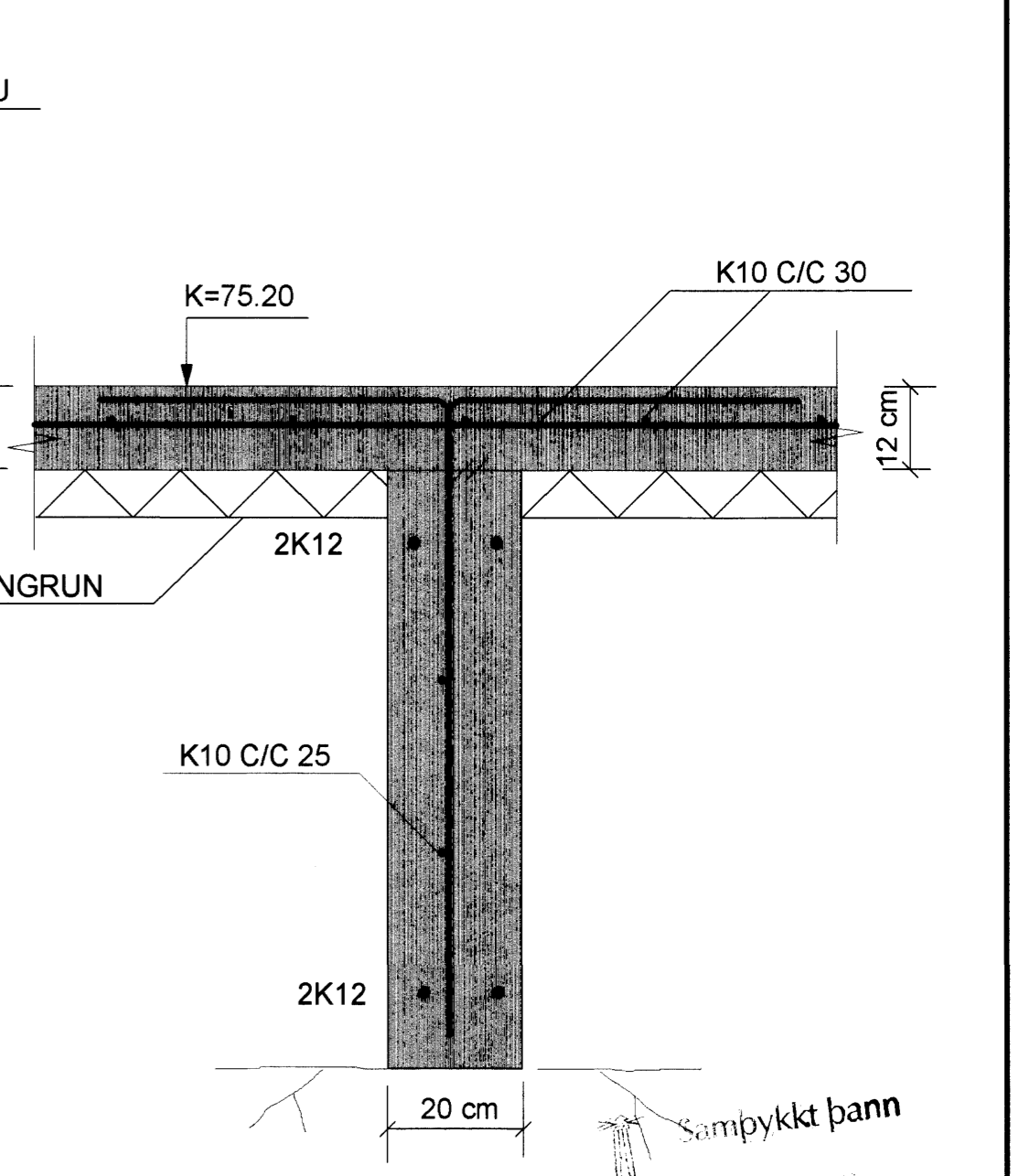
SNID G-G MKV. 1:10
