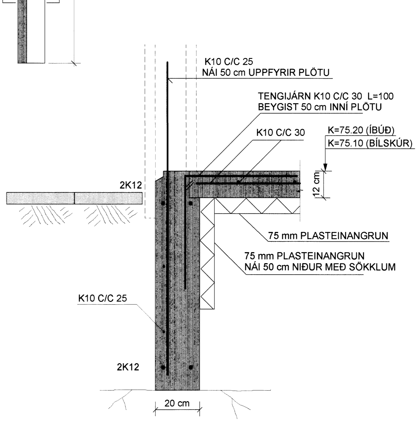
SNID A-A MKV. 1:10
