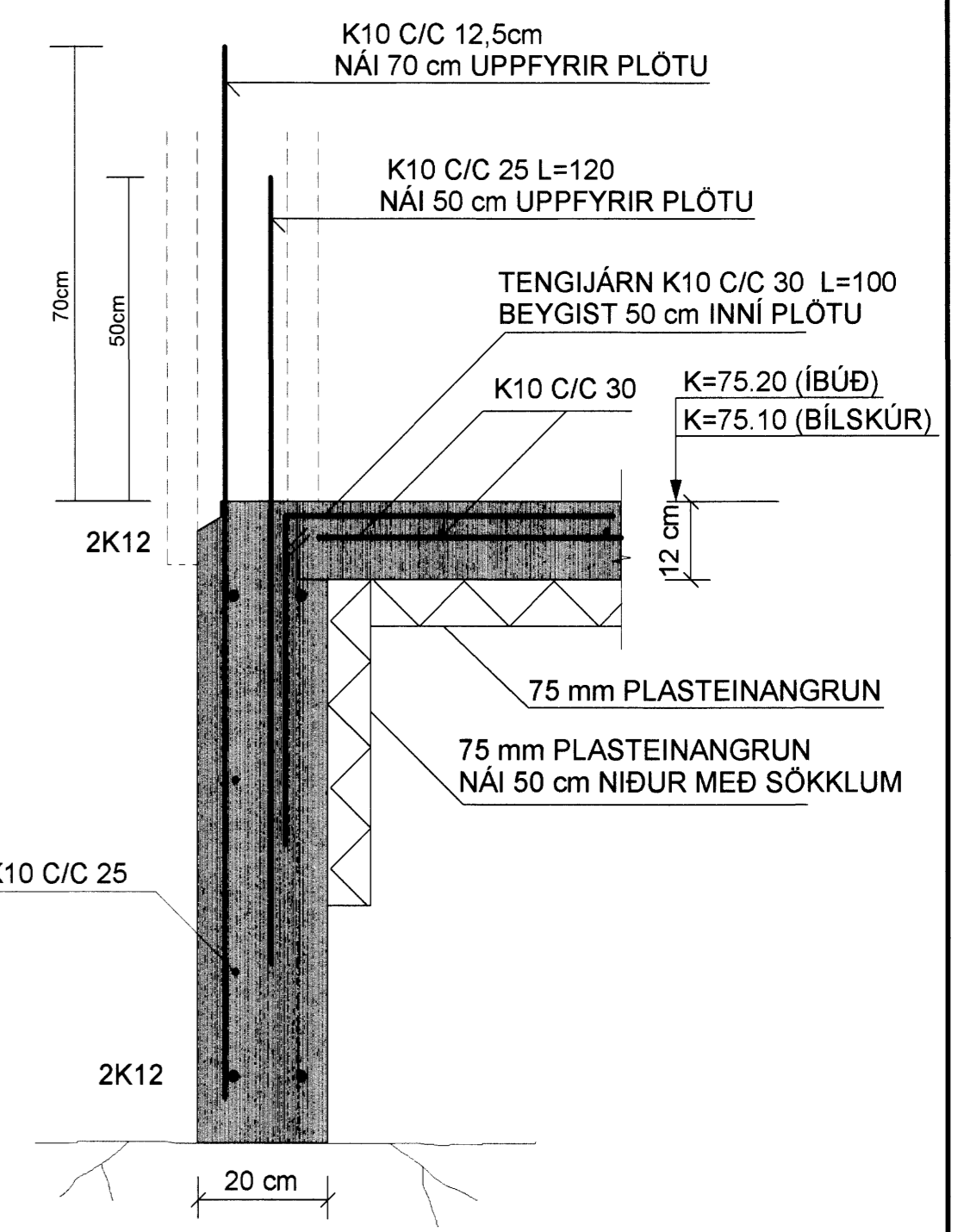
SNID B-B MKV. 1:10
