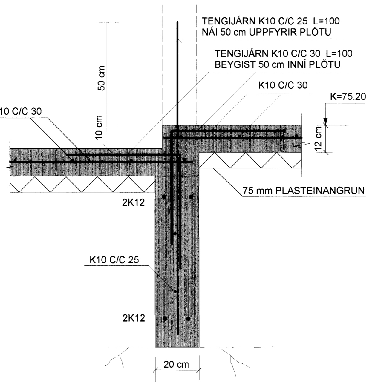
SNID D-D MKV. 1:10
