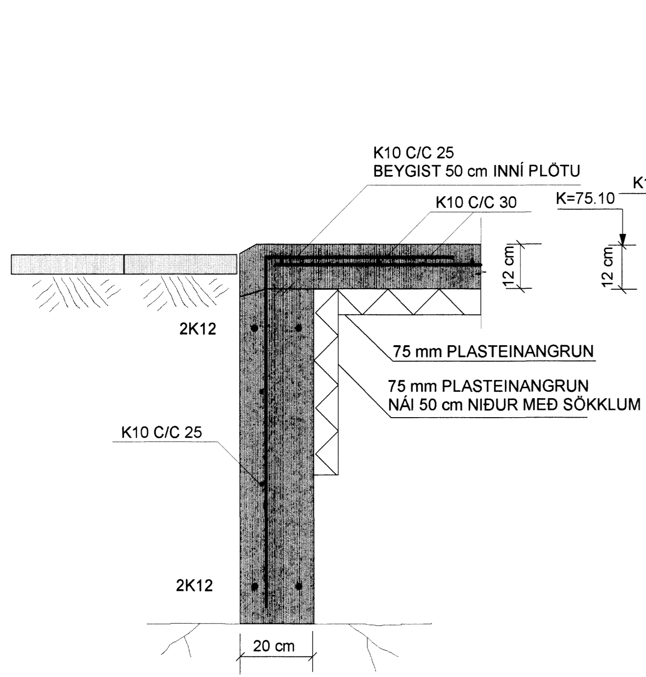
SNID C-C MKV. 1:10
