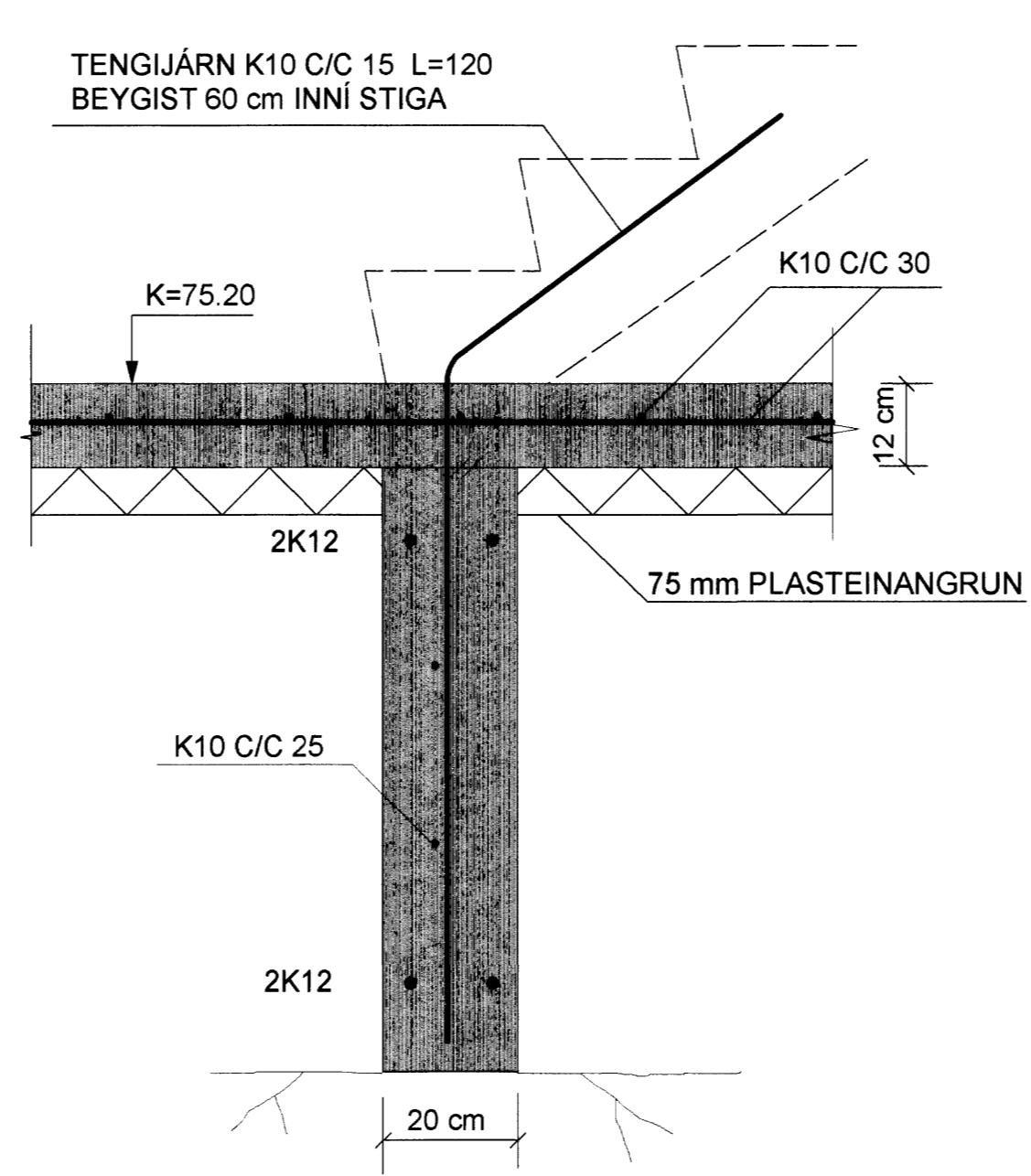
SNID E-E MKV. 1:10
