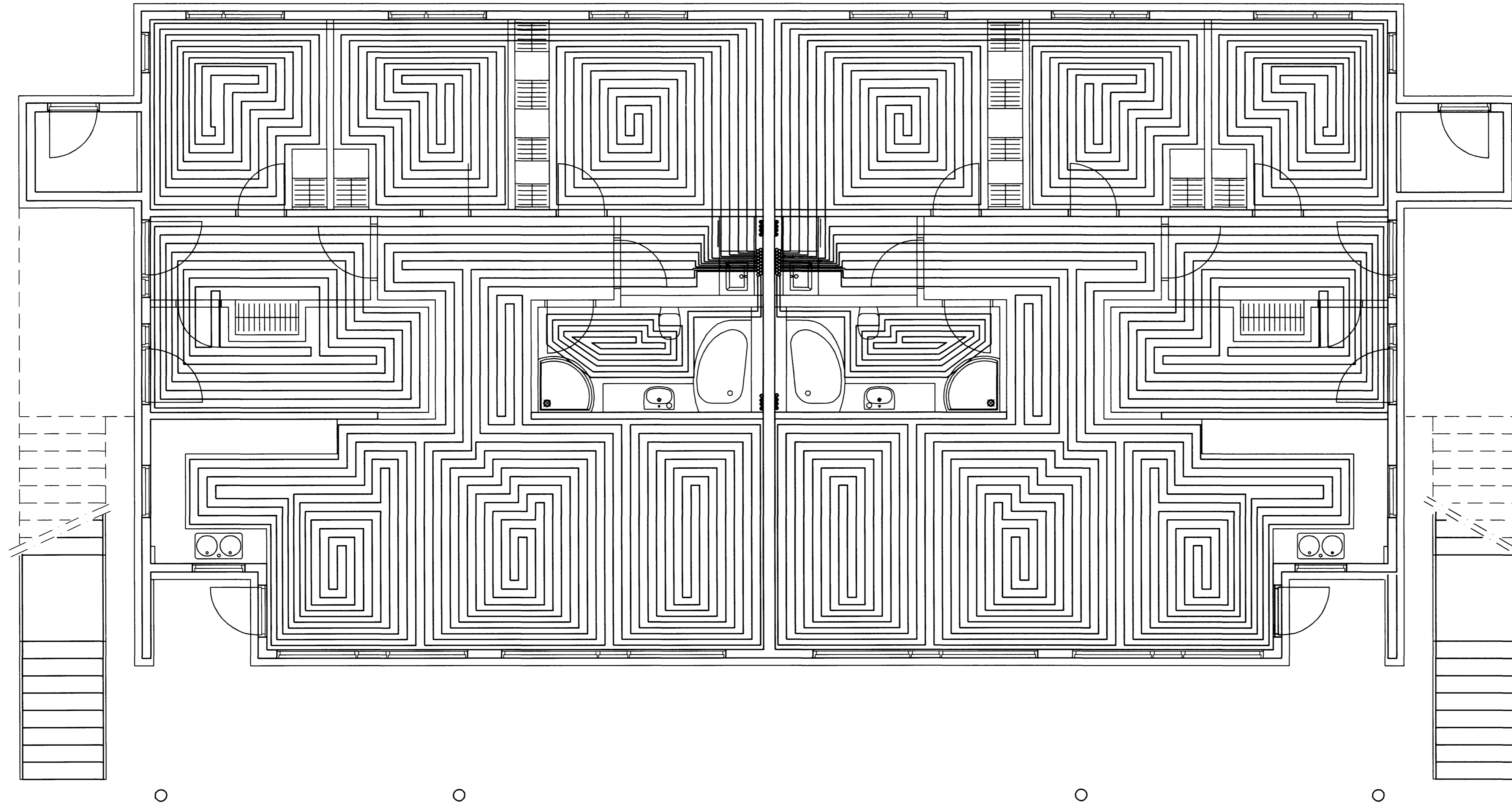
GRUNNMYND 1 HÆÐAR 1:50
