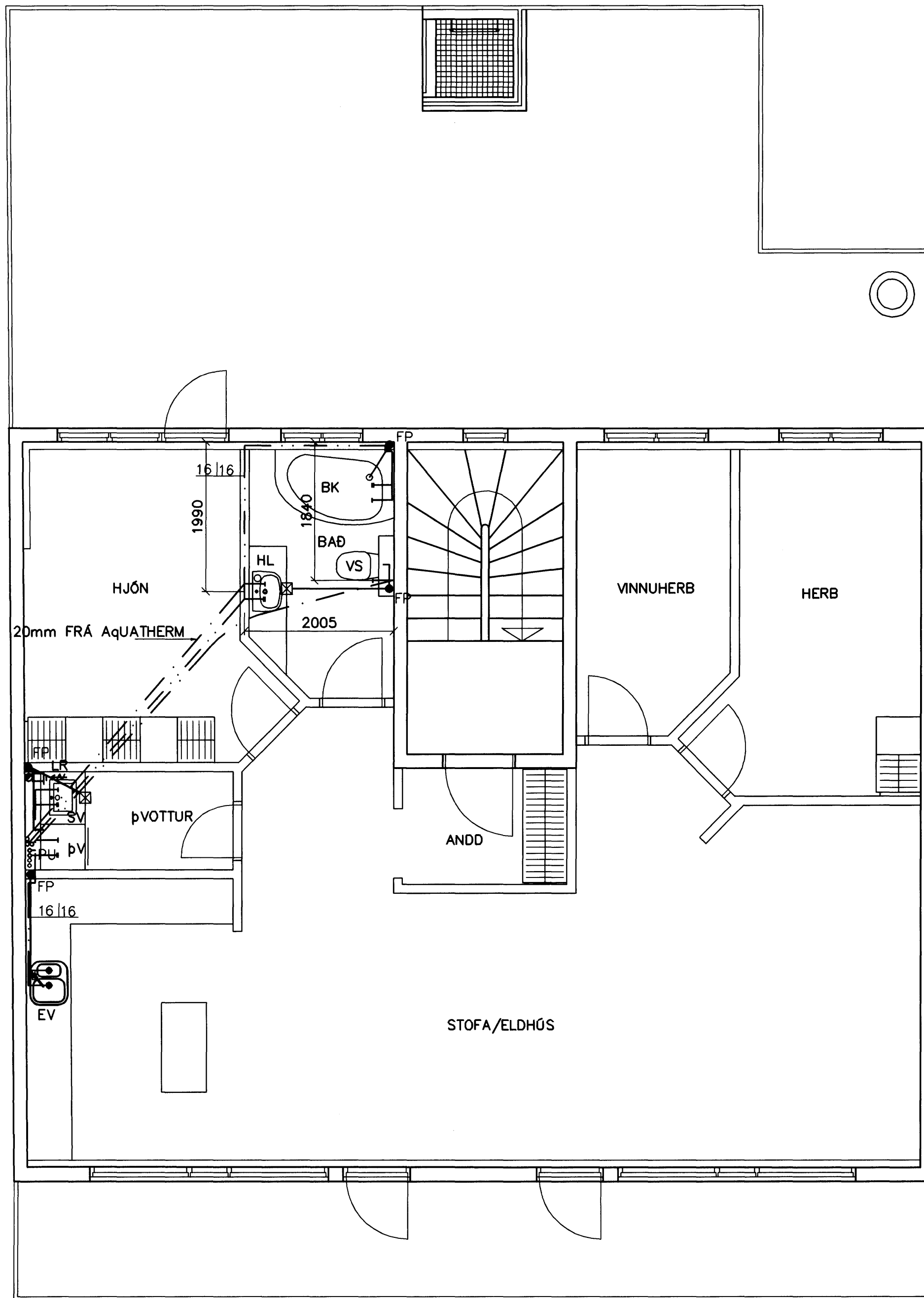
GRUNNMYND 2 HÆÐAR 1:50
