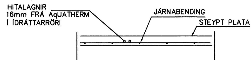
LAGNIR, SNIÐ, 1:20
