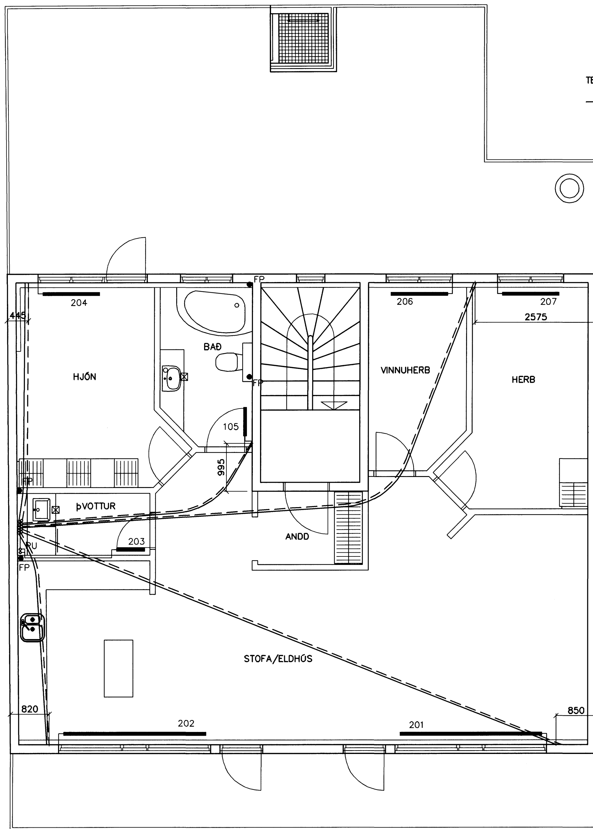
GRUNNMYND 2 HÆÐAR 1:50
