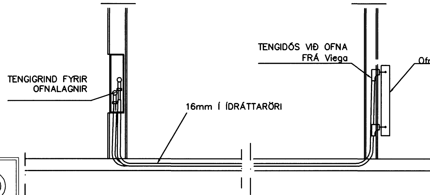
TENGIÐ OFNALAGNALAGNA 1:20
