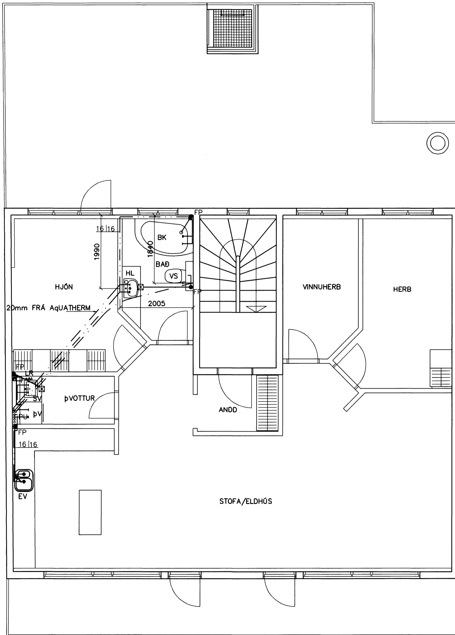
GRUNNMYND 2 HÆÐAR 1:50
