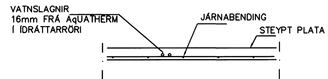
LAGNIR, SNIÐ, 1:20
