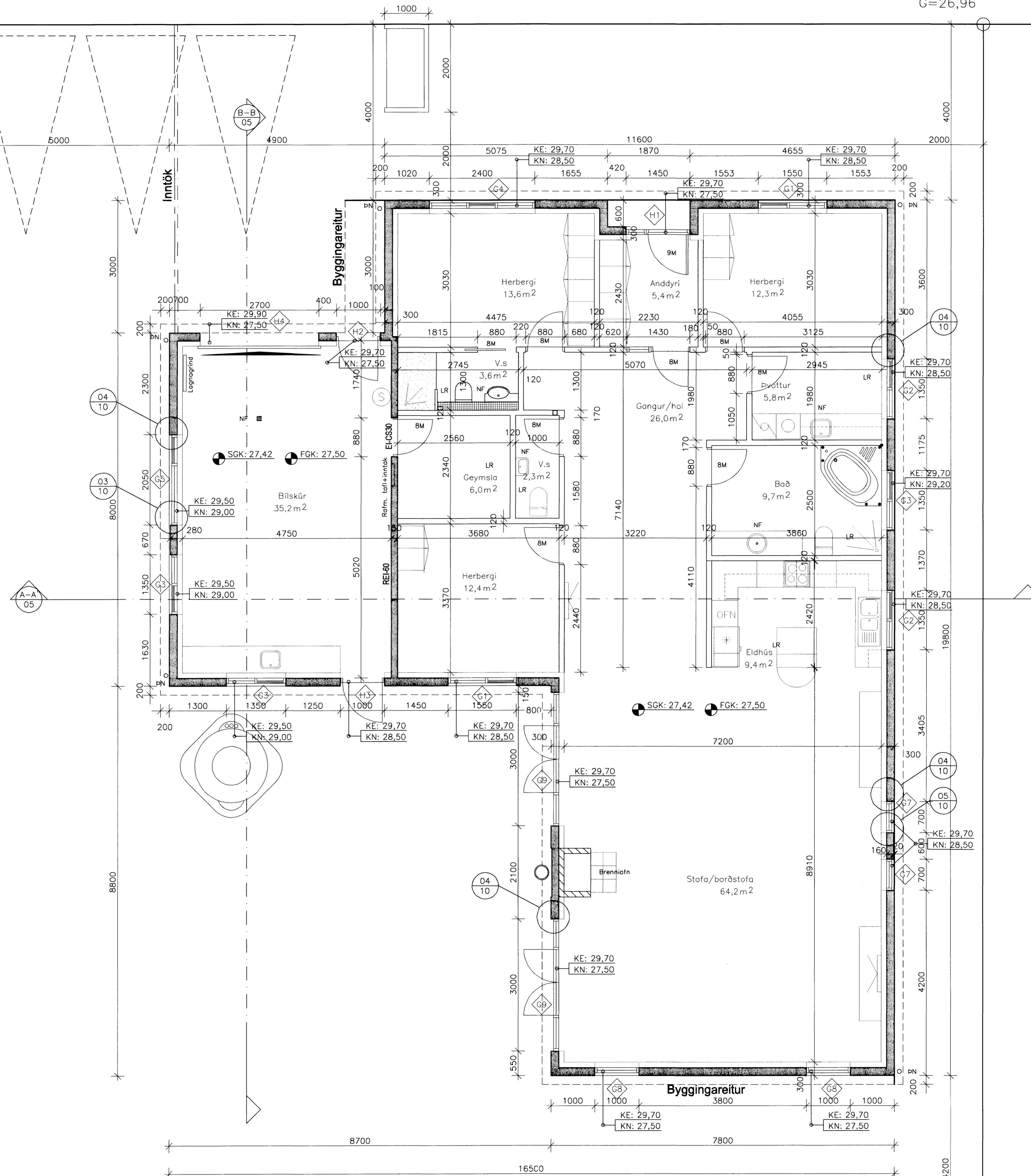
GRUNNMYND 1. HÆÐAR 1:50
