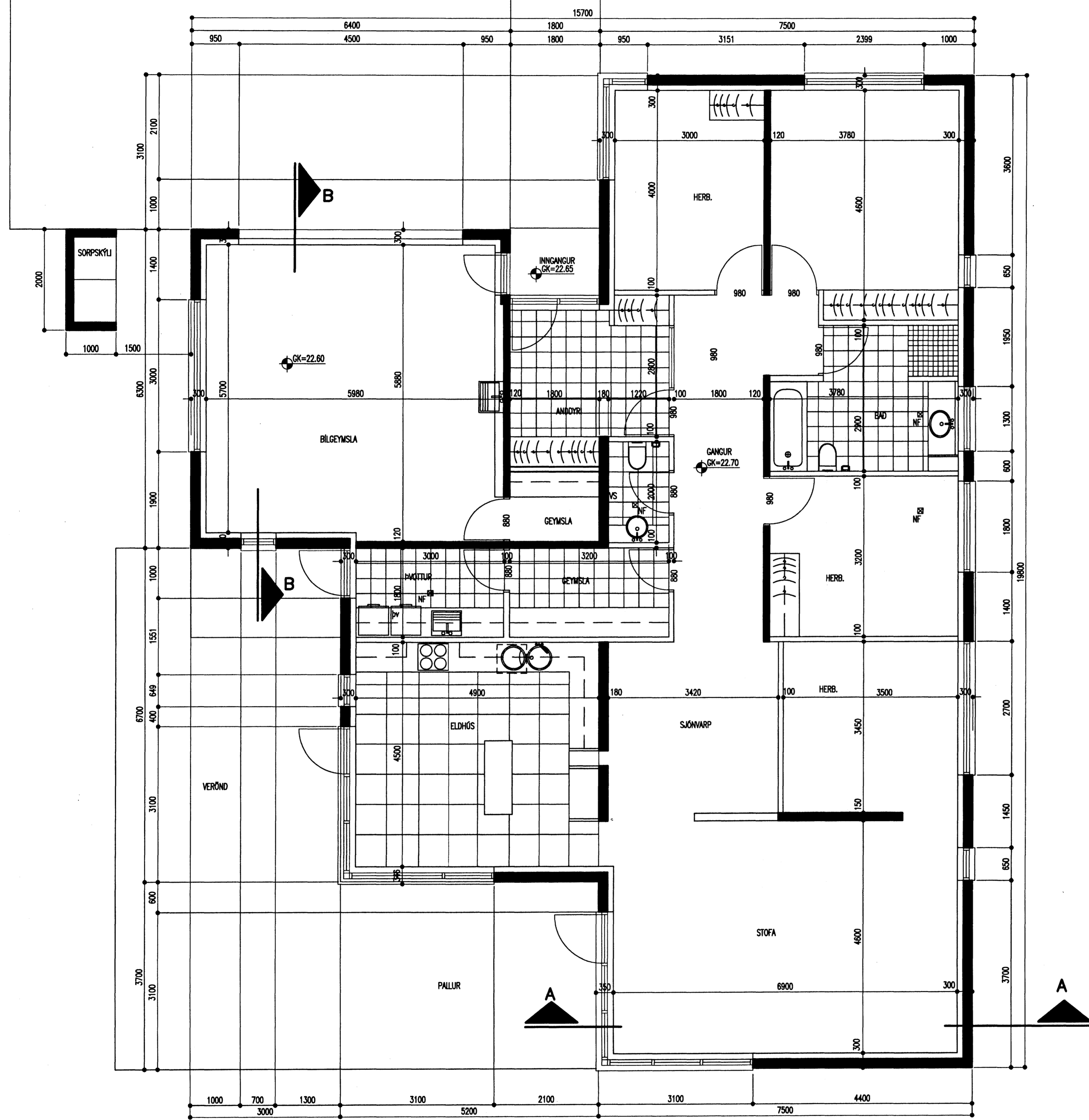
GRUNNMYND – MKV 1:50
