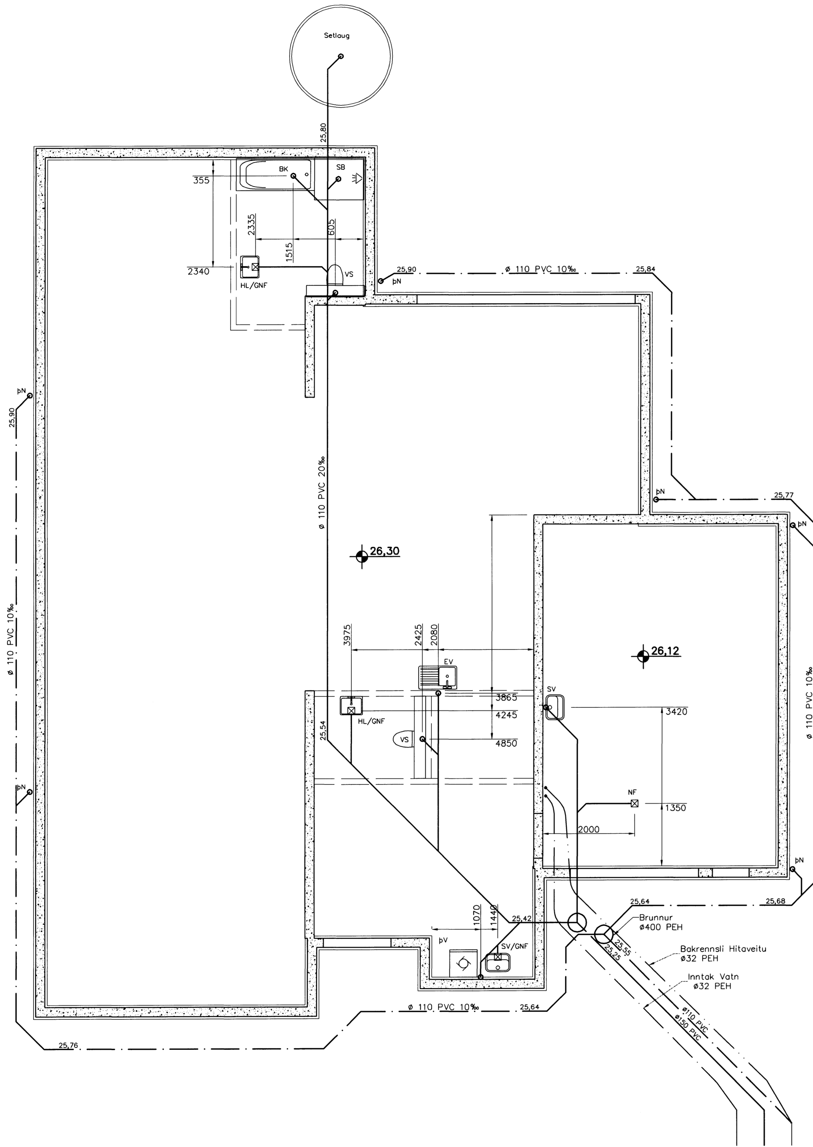
Grunnlagnir 1:50
