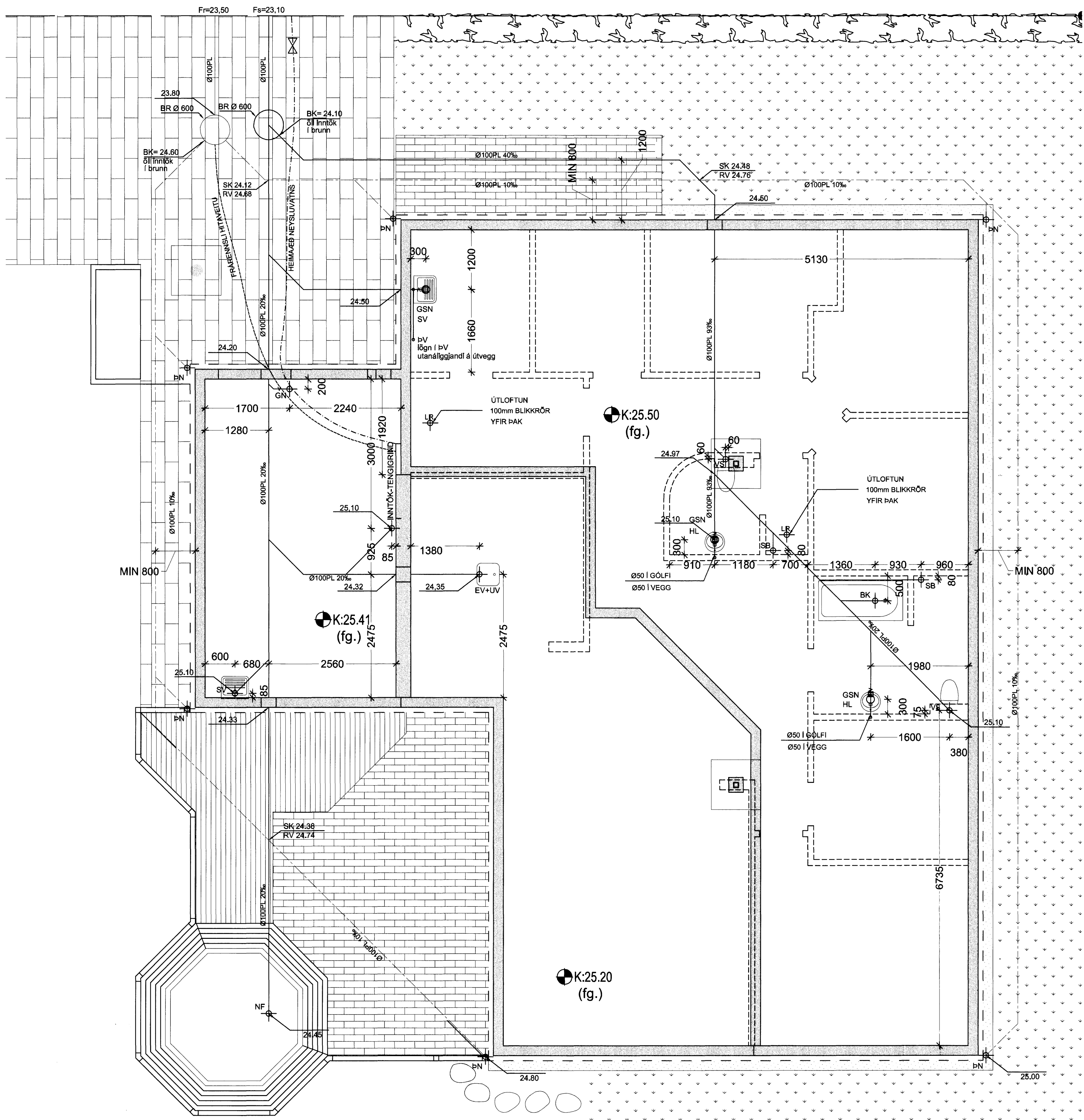
AFSTÖÐUMYND MKV. 1:500
