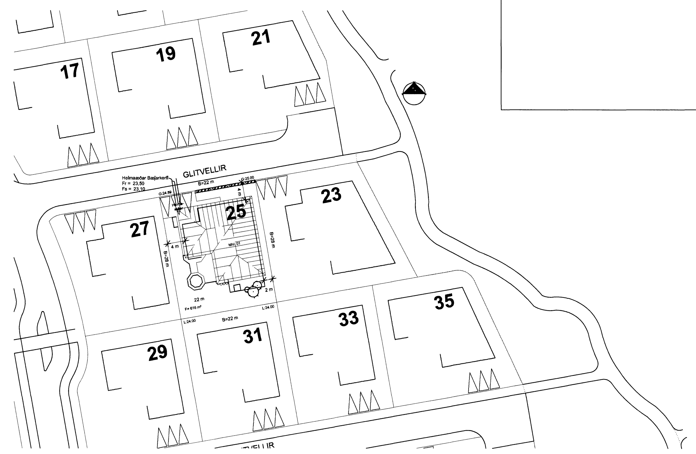
AFSTÖÐUMYND MKV. 1:500
