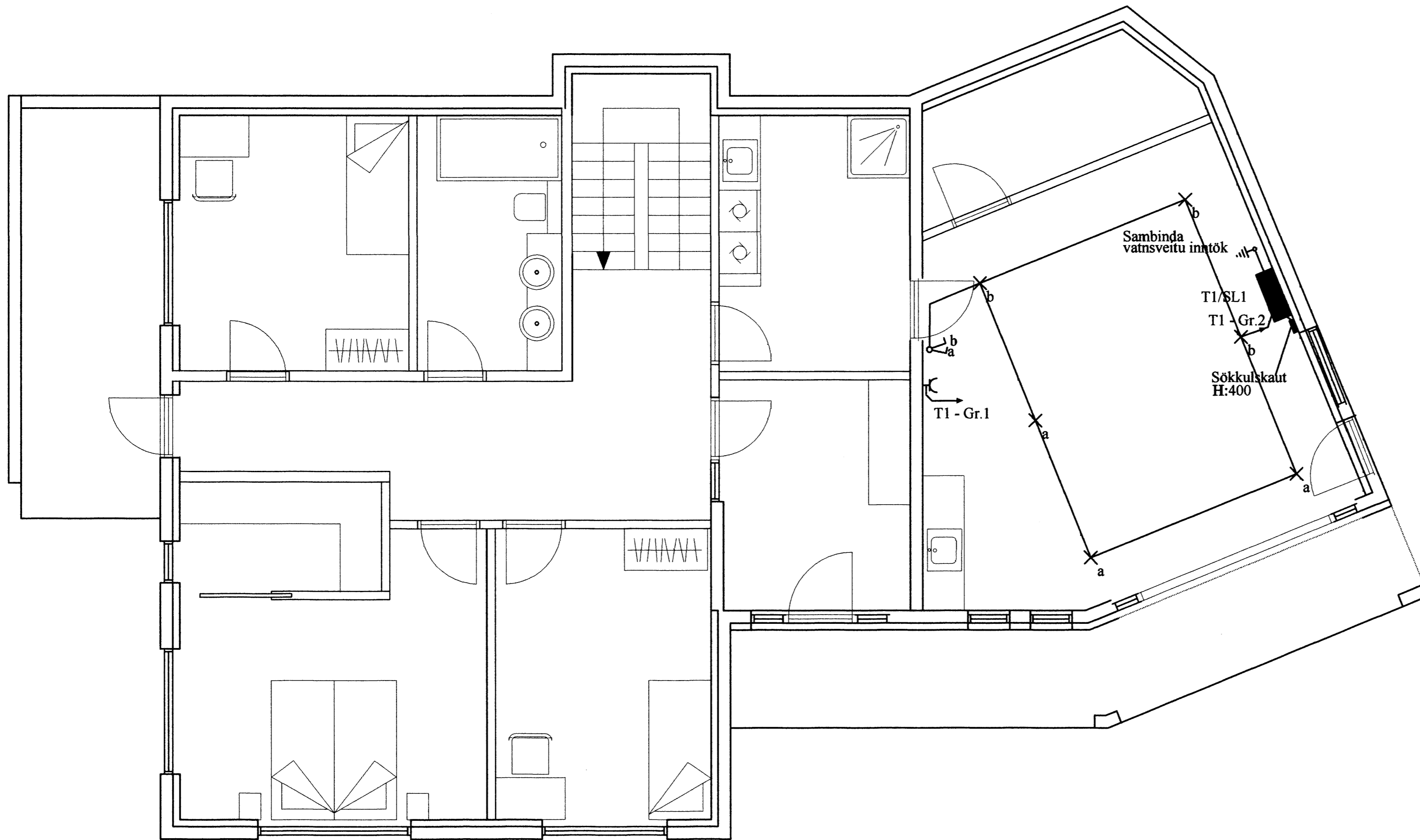
Grunnmynd - Raflögn neðri hæðar
