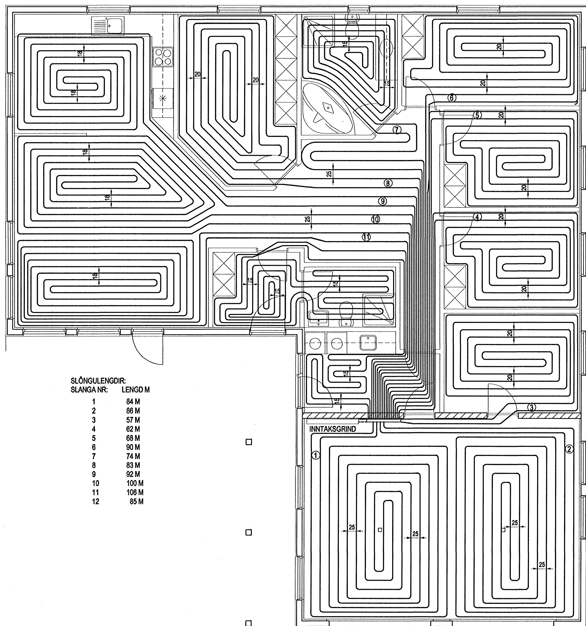
GÓLFHITALAGNIR - GRUNNMÝND MKV. 1:50
